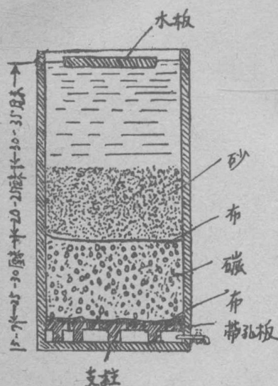
图5 砂炭滤水器
