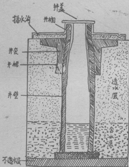
图1 合理修建的水井
