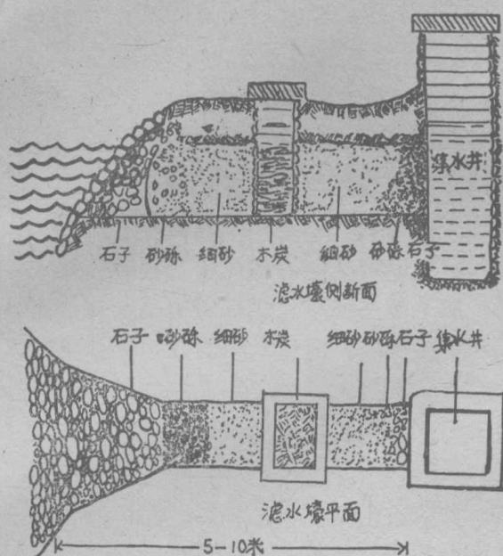
图3 滤水壕
