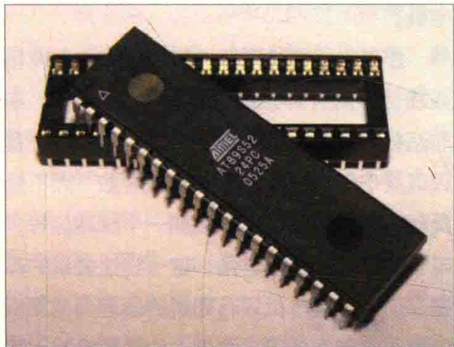
■ 图 1.2 单片机可以作为机器人的控制芯片
