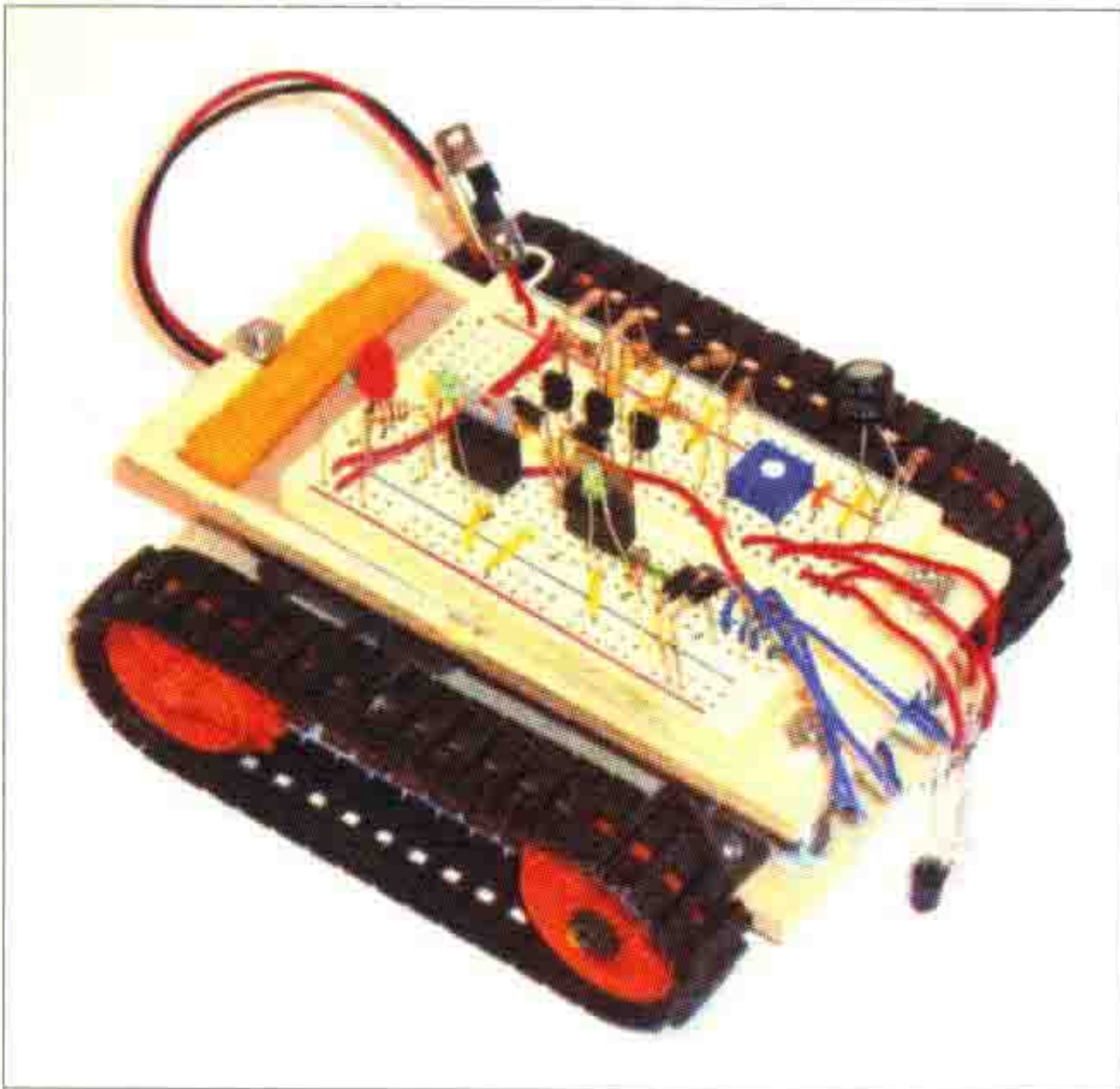
图 1.8 用面包板也能做出机器人小车
