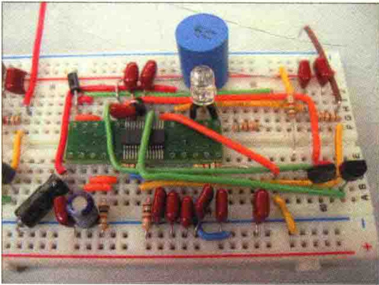
图 1.7 面包板可以方便地修改电路
