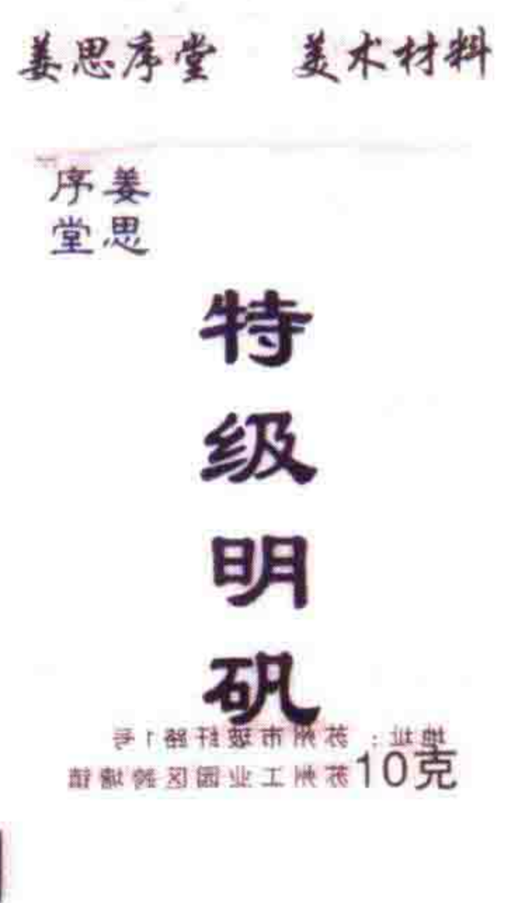
明矾
