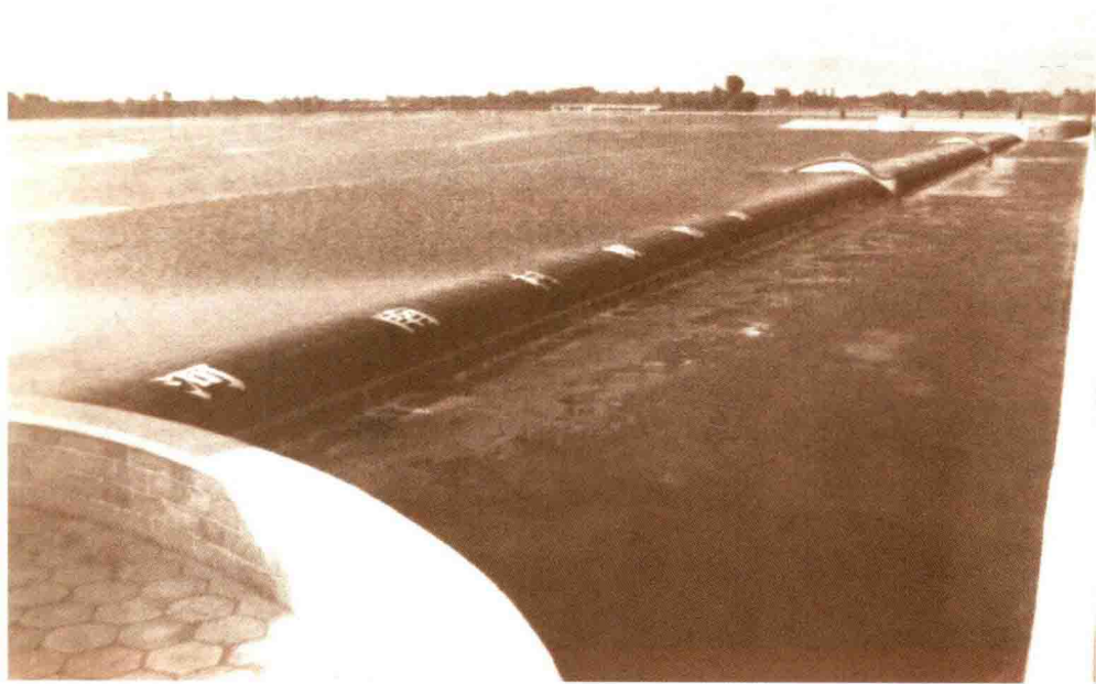
1992 年修建的潮白河河南村橡胶坝
