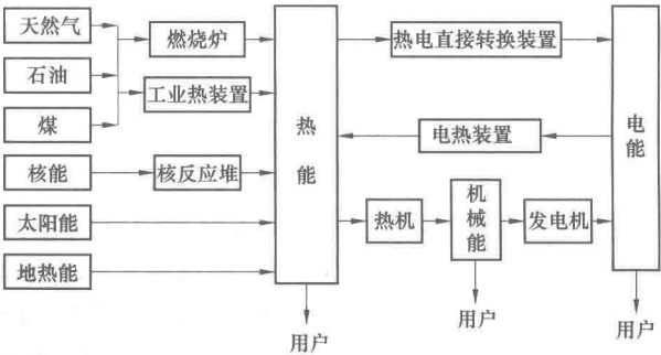
图 1-1 不同能源与热能的转换及利用情况
