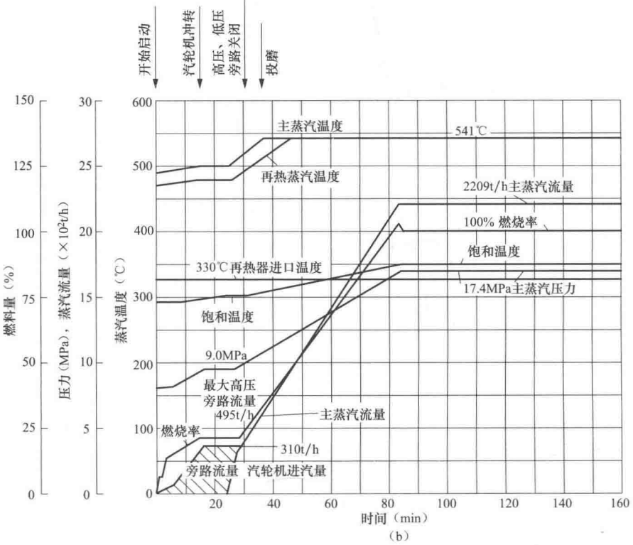
图 1-4 某 2208t/h 亚临界自然循环汽包炉热态和极热态滑参数启动曲线 (a) 热态启动; (b) 极热态启动
