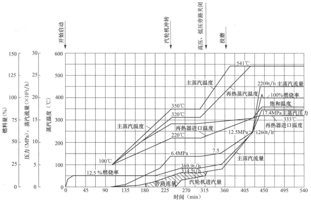
图 1-3 某 660MW 亚临界机组 2208t/h 自然循环锅炉的冷态滑参数启动曲线
