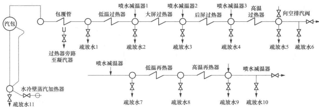
图 1-1 自然循环汽包锅炉典型汽水系统与疏放水系统
