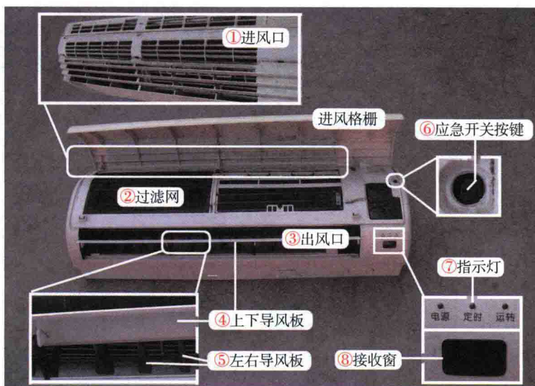
图 1-9 室内机正面结构
