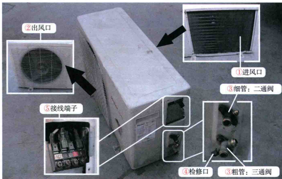
图 1-11 室外机外部结构
