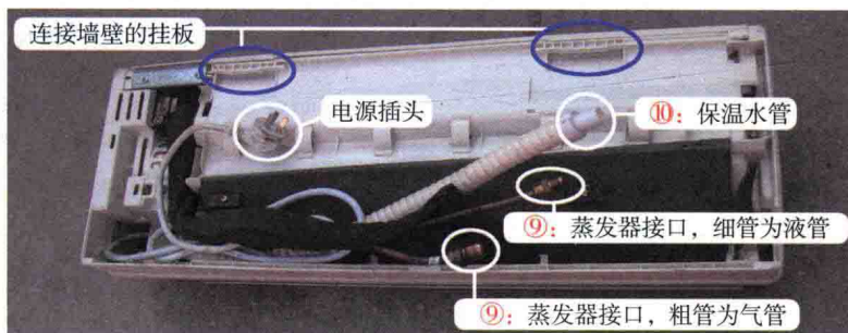
图 1-10 室内机反面结构
