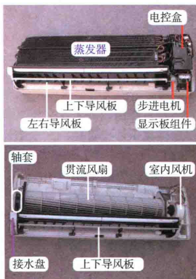
图 1-13 室内机主要部件
