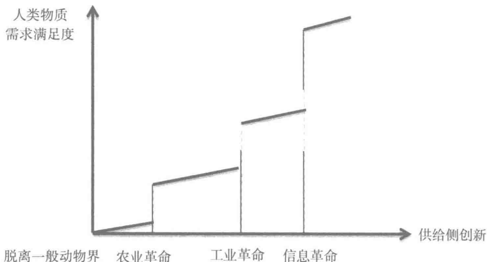
图1 供给侧创新作用原理的量化表达（阶跃量化曲线）
