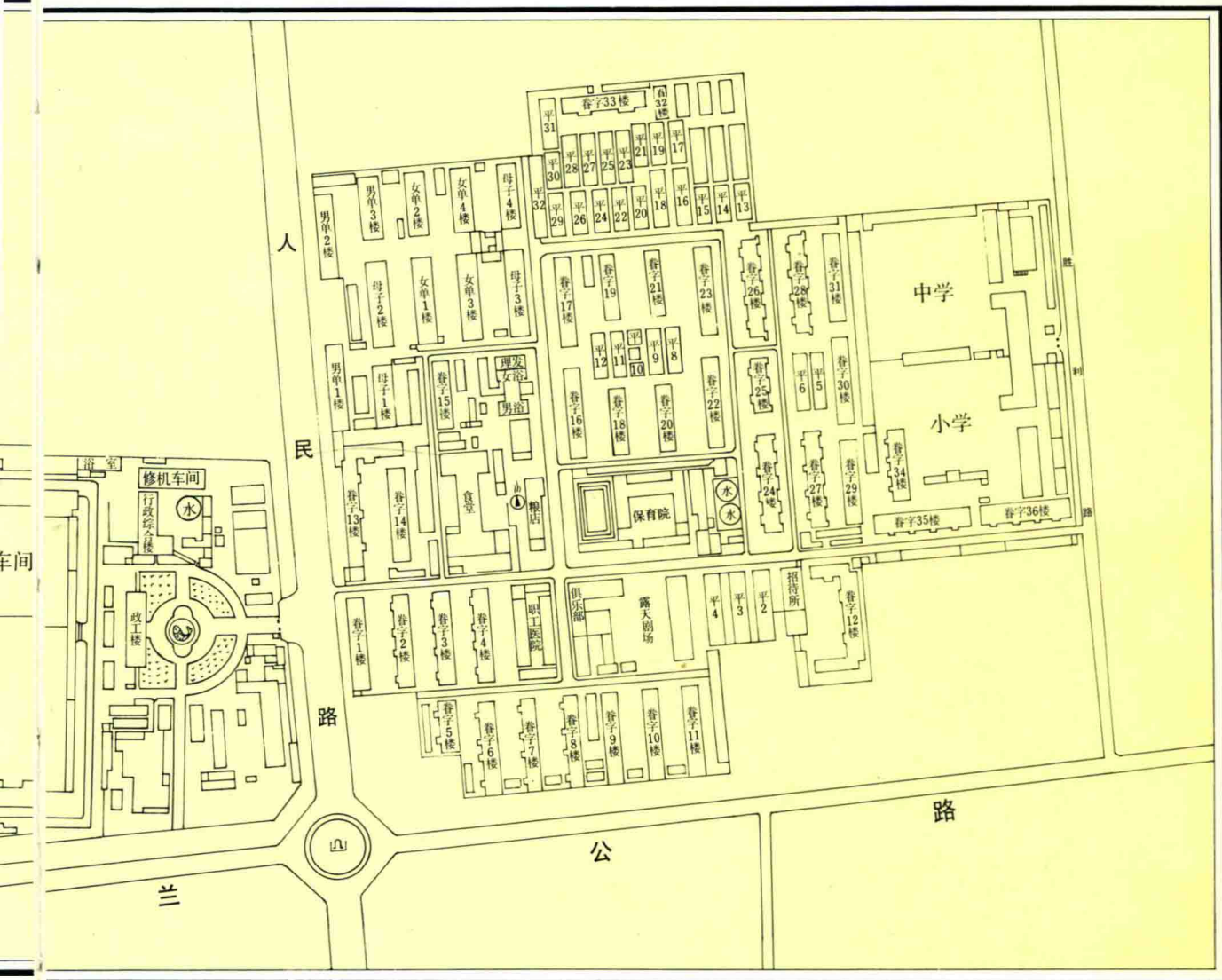
棉纺织厂总平面图
