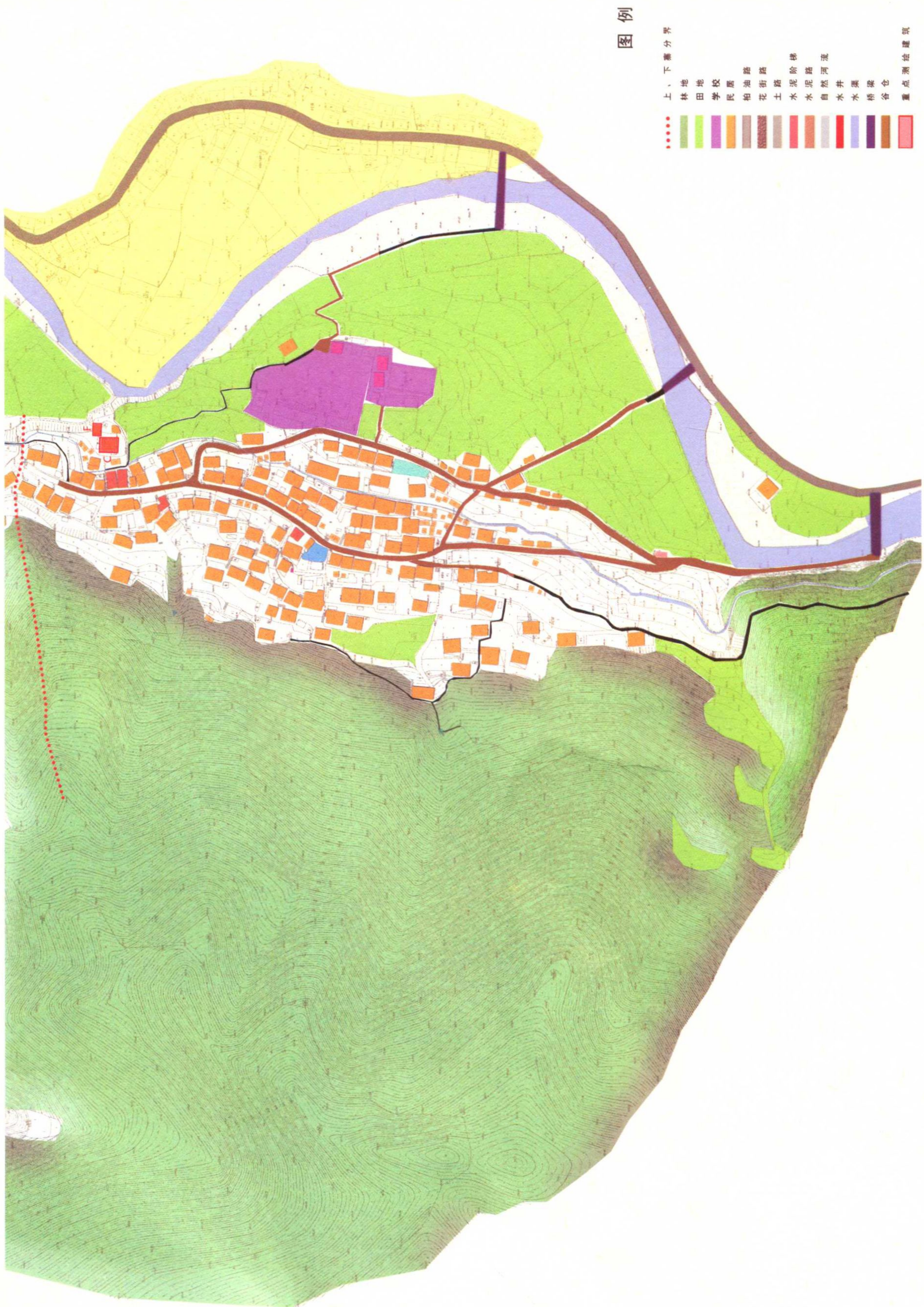
卡寨村图版五 卡寨下寨总平面图
