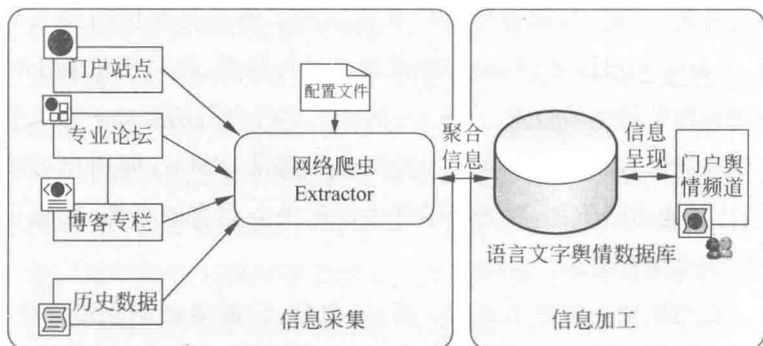
图1 语言文字网络舆情自动监测示意图
