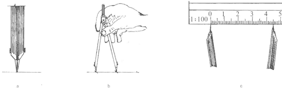
图 1-5 分规的用法
