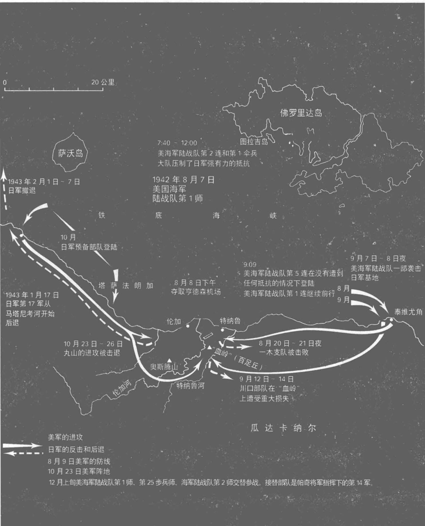
★ 1942年8月~1943年2月，美、日军队在瓜达卡纳尔岛战役中重要军事行动示意图。
