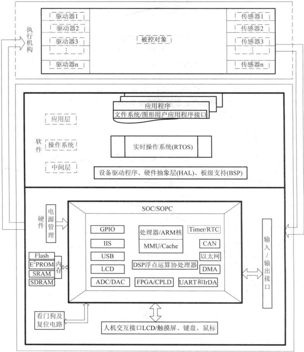
图 1.2 基于控制领域的典型嵌入式系统
