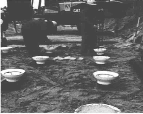
图 1-7 安置塑料套管模具及放置钢筋
