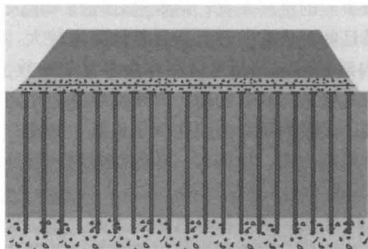
图 1-1 桩承式加筋路堤
