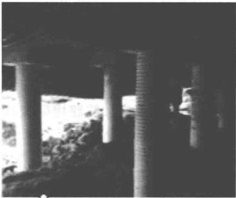
图 1-4 使用阶段 AuGeo 桩
