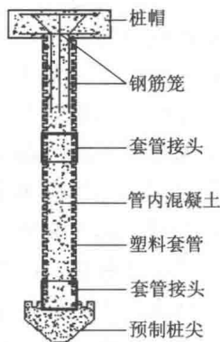
图 1-2 TC 桩组成示意
