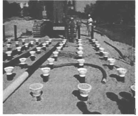
图 1-8 集中浇筑混凝土
