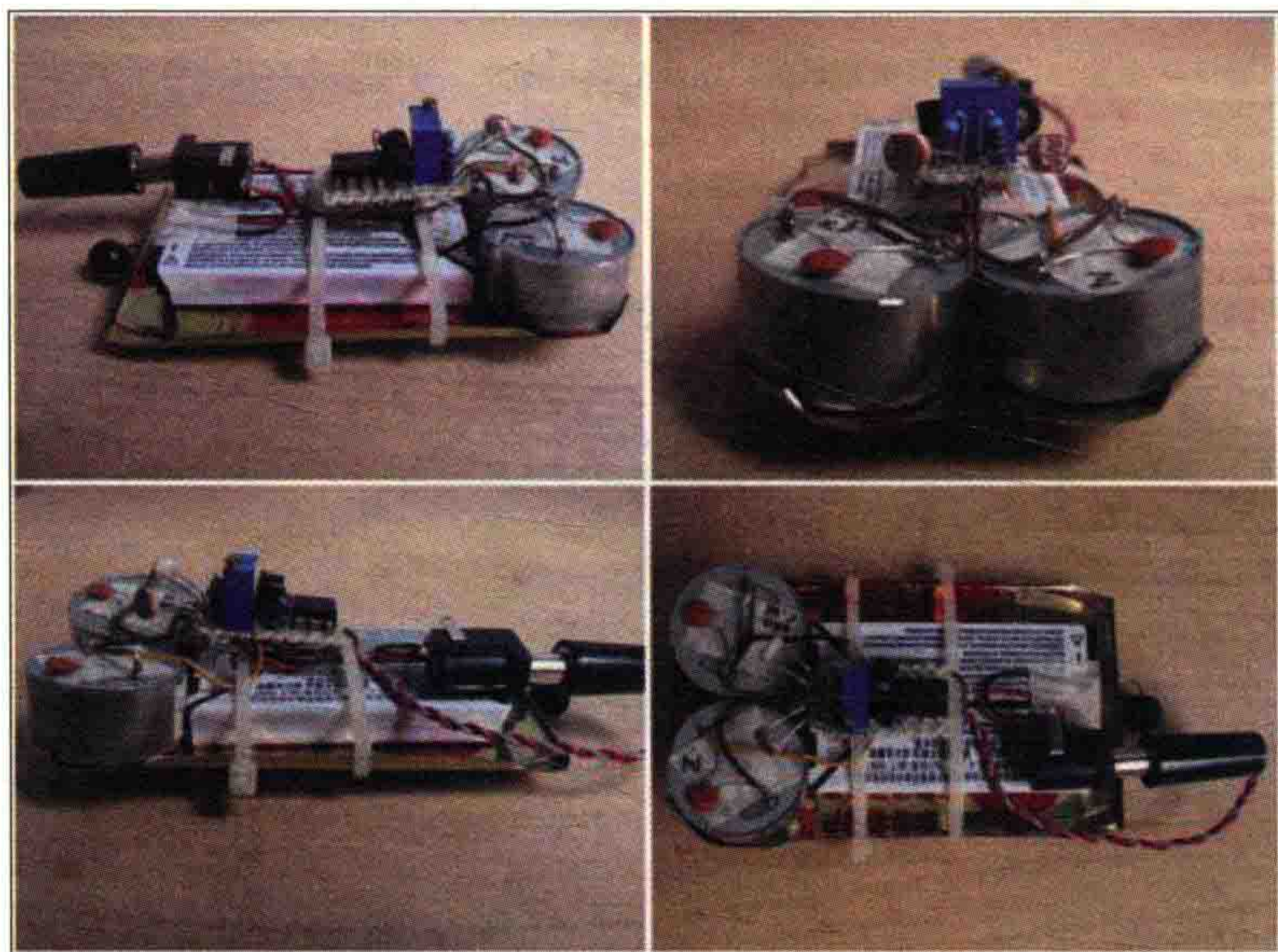
图 1-5 业余制作可以尽情发挥创意，使用任何可以利用的材料。这是一个以铁罐头皮为底盘制作的寻光机器人。两只电机固定在底盘上，尾轮是一个塑料珠子，电源是淘汰下来的手机电池，电子部分焊在一小块洞洞板上，用尼龙扎带把这些捆绑在一起，就构成了一个智能移动平台，是不是很有趣？
