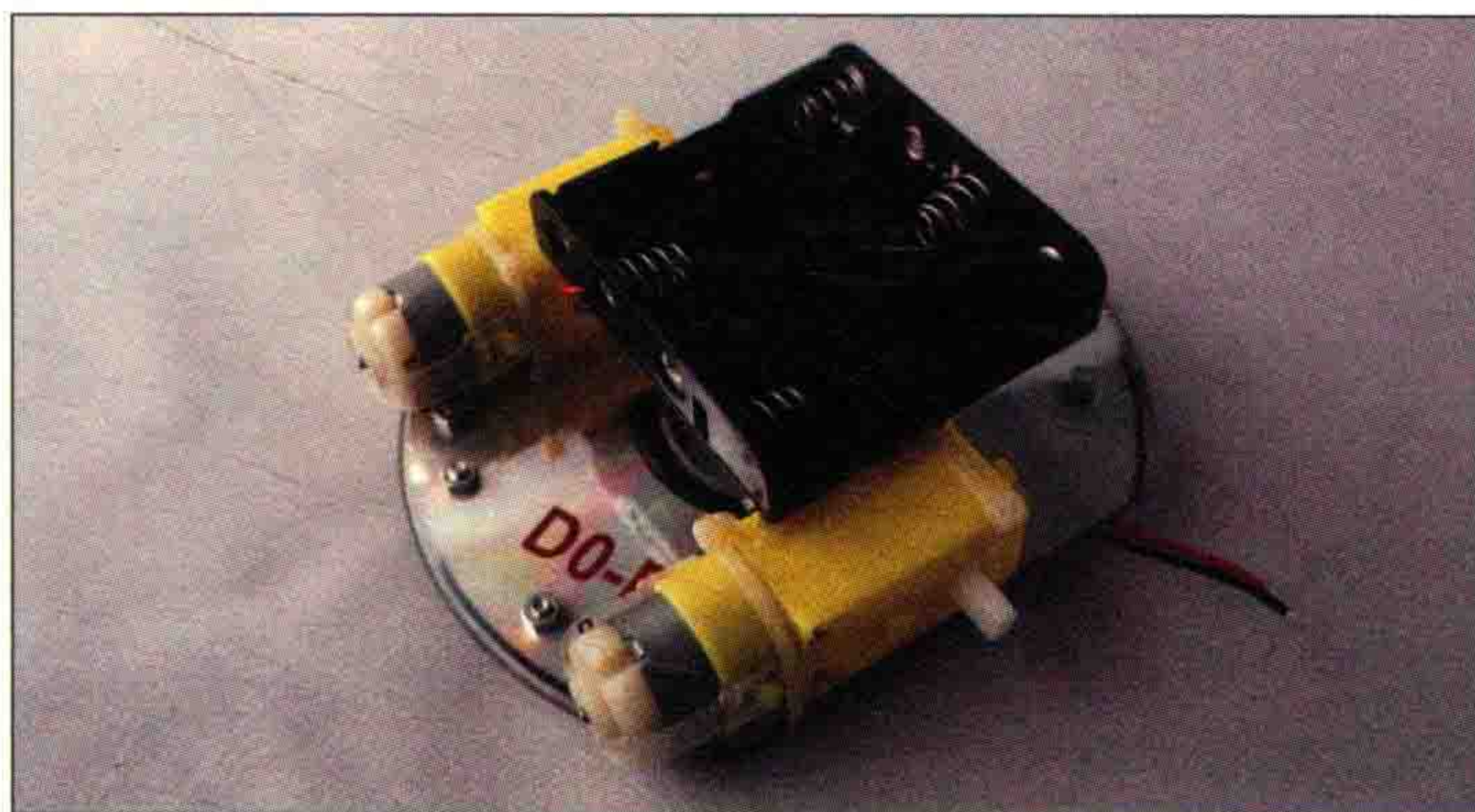
图1-11 把两片光盘叠起来，用M3螺丝固定好，电机和电池盒用尼龙扎带和热熔胶固定
