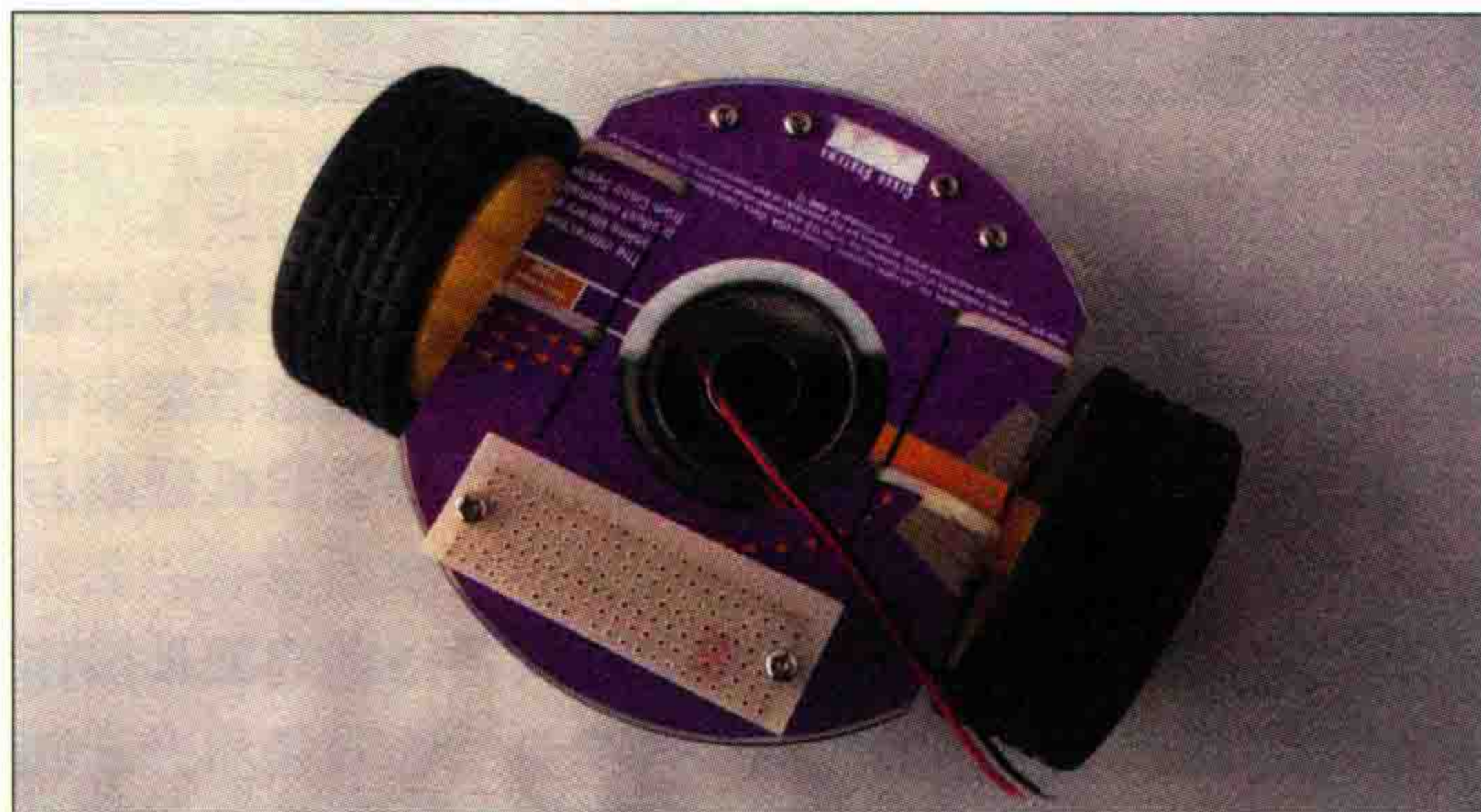
图1-12 车轮插接在电机上，洞洞板用铜柱固定在顶板上
