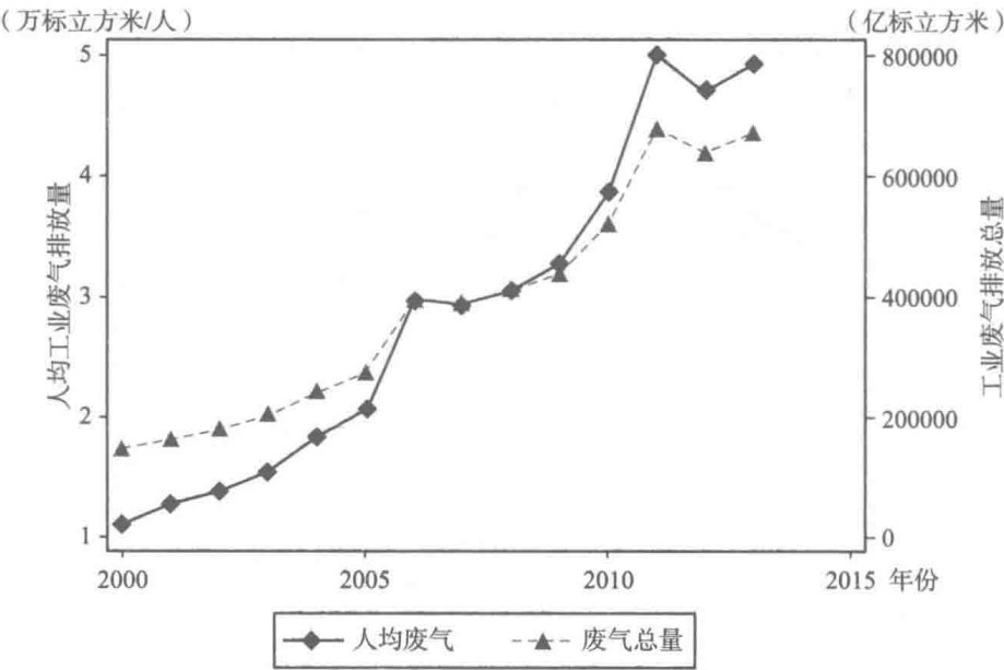
图 1-2 2000~2013 年工业废气排放总量以及人均工业废气排放量
