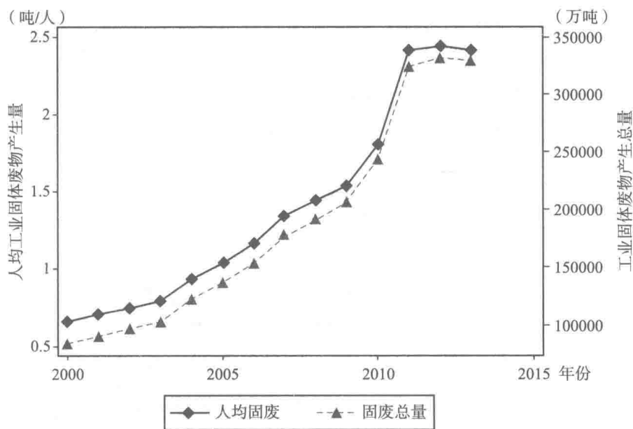
图 1-3 2000 ~ 2013 年工业固废产生总量以及人均工业固废产生量
