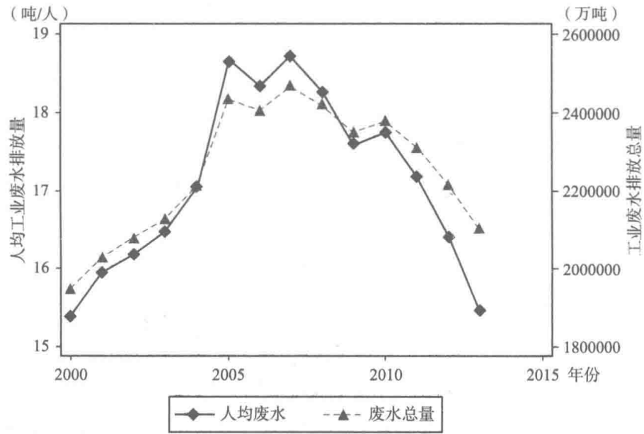
图 1-1 2000~2013 年工业废水排放总量以及人均工业废水排放量
