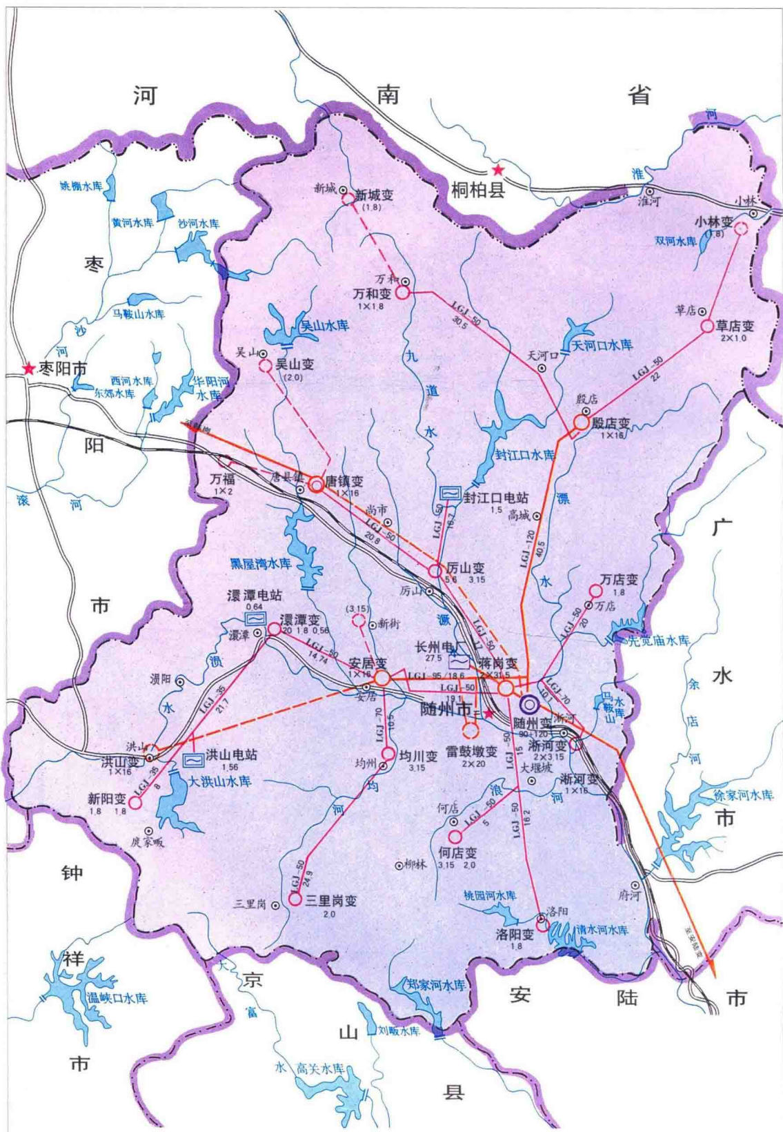
随州市电网地理接线图
