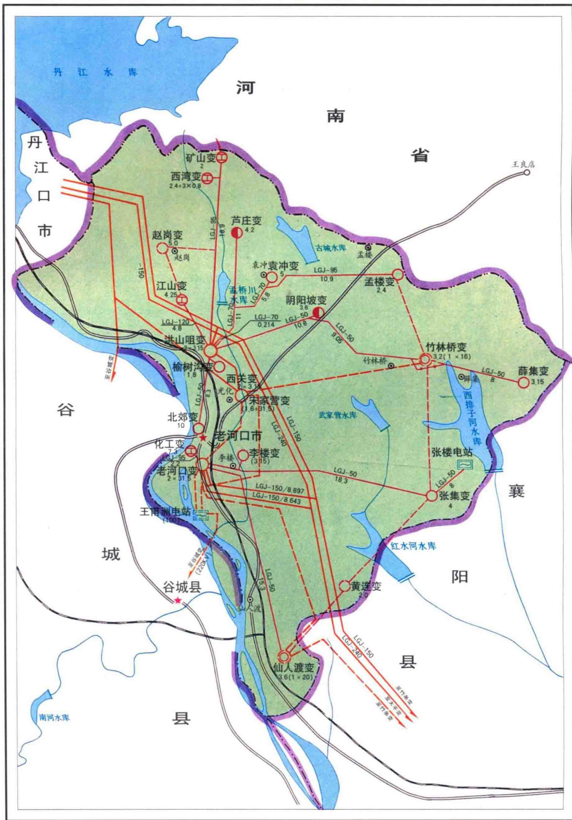
老河口市电网地理接线图
