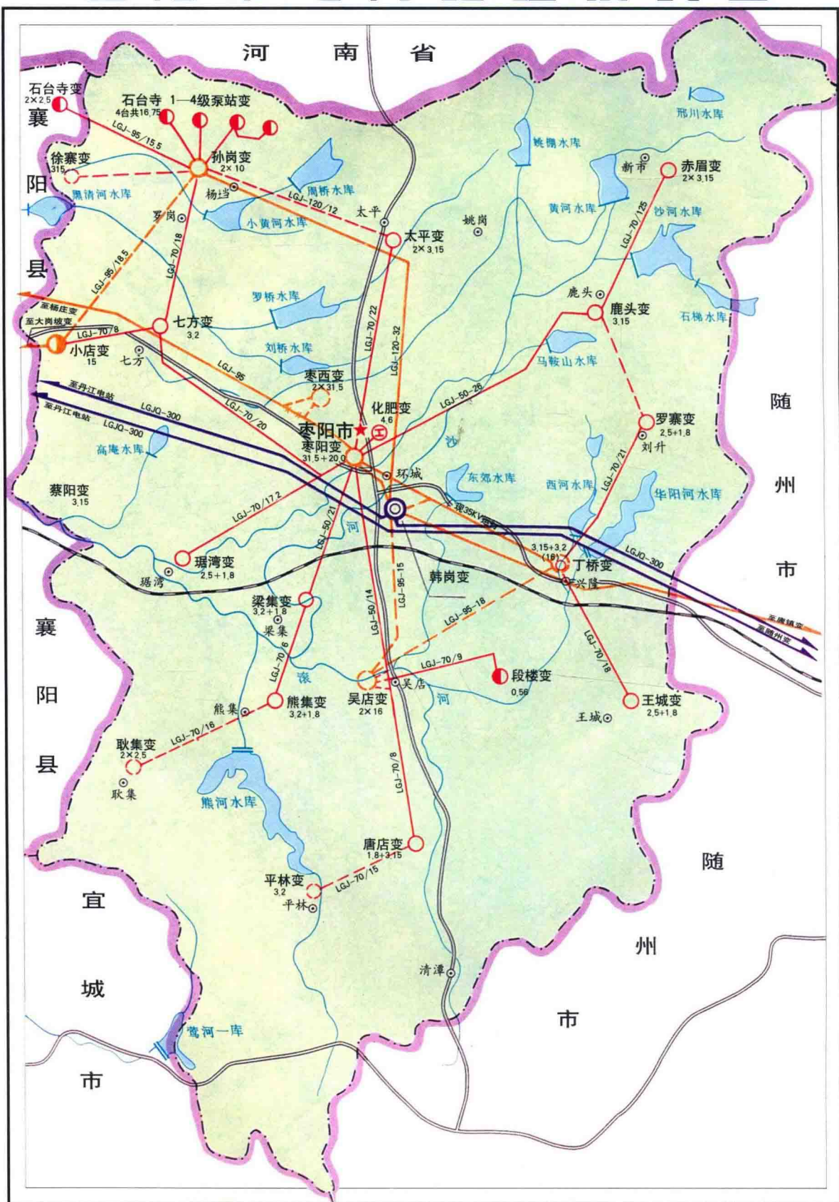
枣阳市电网地理接线图
