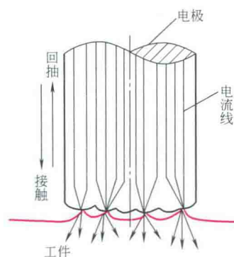
图 1-2 接触引弧示意图
