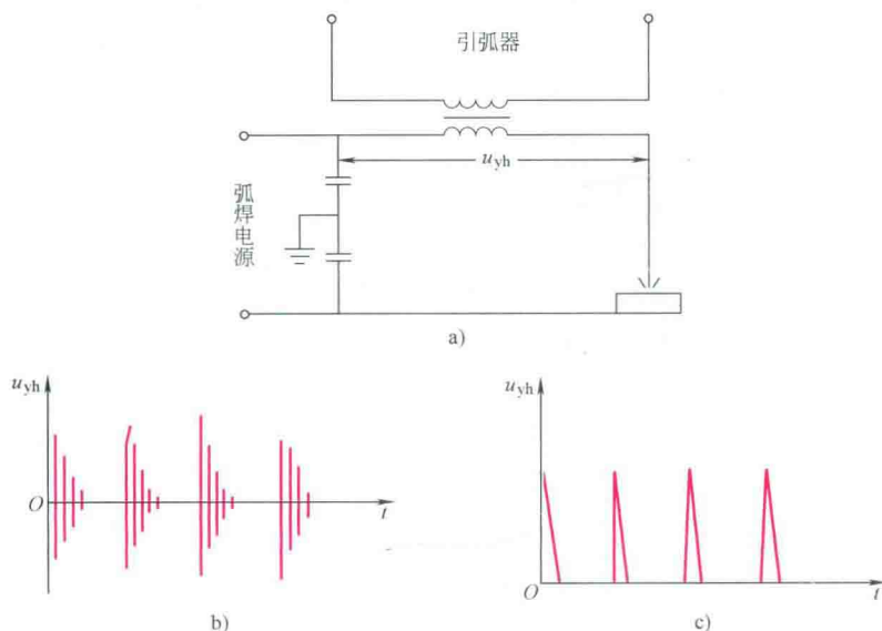
图 1-3 高频高压引弧和高压脉冲引弧示意图
