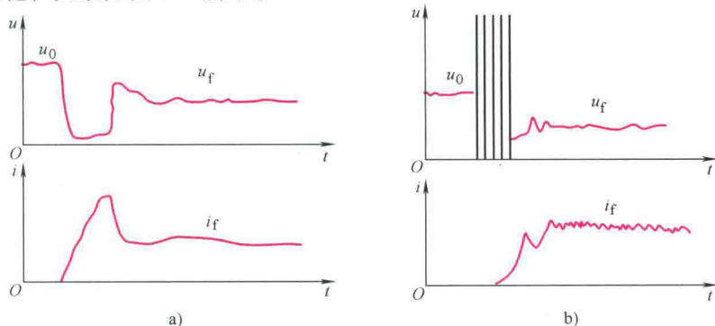
图 1-1 引弧过程的电压、电流变化曲线图
