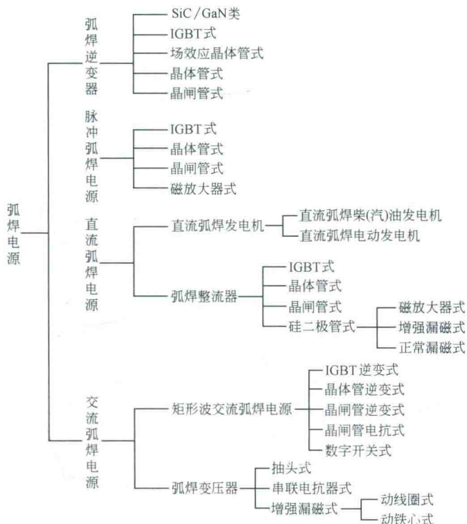
图 0-1 弧焊电源的分类
