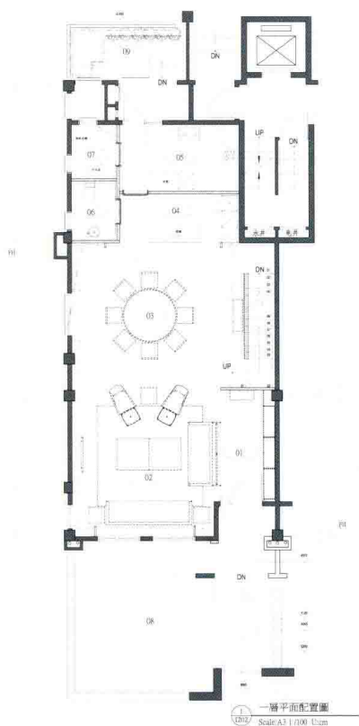
一层平面图
