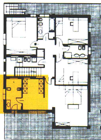
二层平面图
