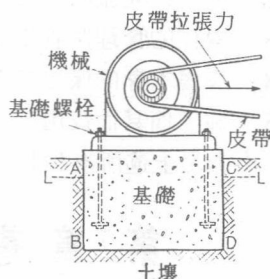
圖 2-1 基礎周圍有支持土壤的機械基礎一例
