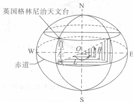
图 1-3 参心坐标系
