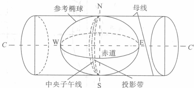
图 1-4 高斯直角坐标系的投影图
