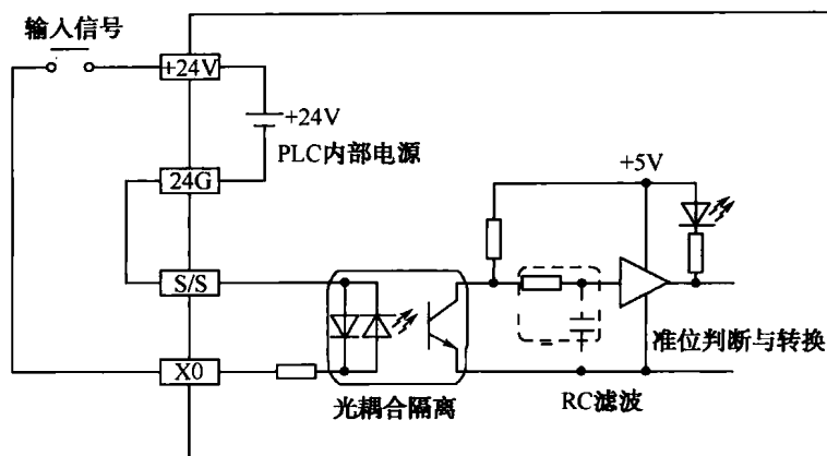
图 1-1 输入信号图
