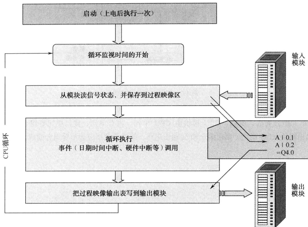
图 1-3 PLC 的工作过程图
