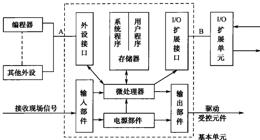
图 1-2 PLC 基本结构框图
