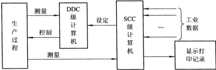
图 1-1-5 计算机监督控制系统结构图
