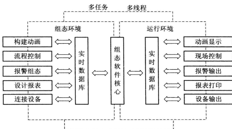
图 1-1-9 MCGS 工控组态软件的整体结构
