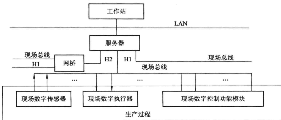
图 1-1-8 现场总线控制系统结构图
