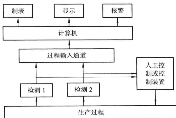
图 1-1-3 计算机数据采集系统结构图
