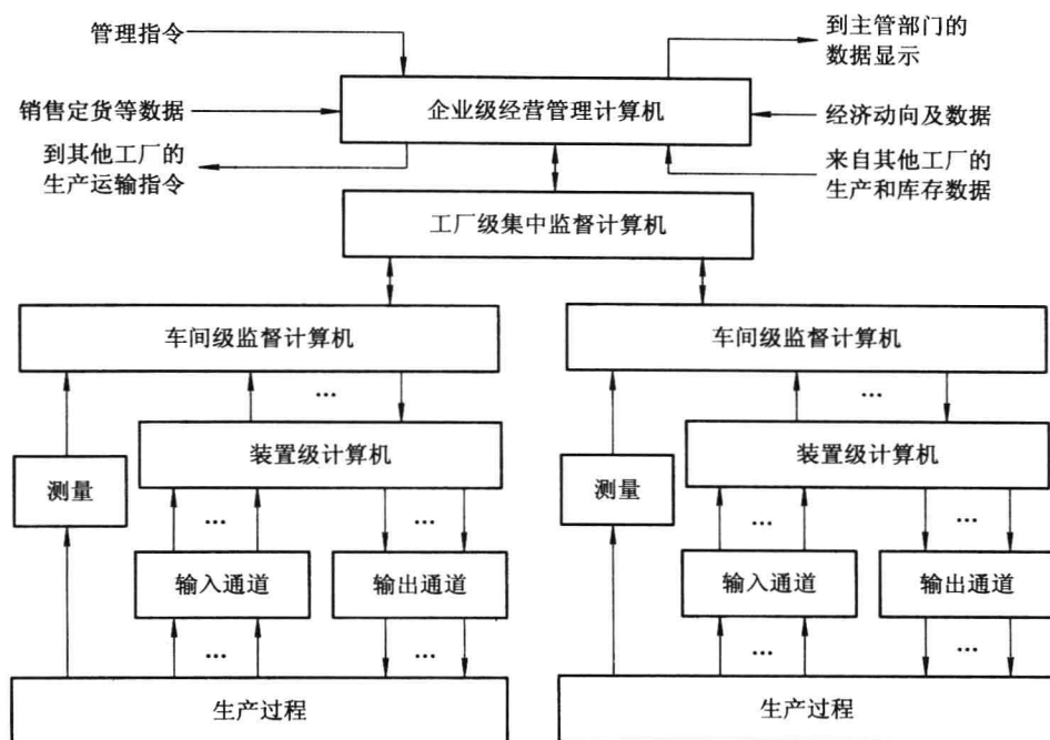
图 1-1-6 四级的计算机分级控制系统结构图
