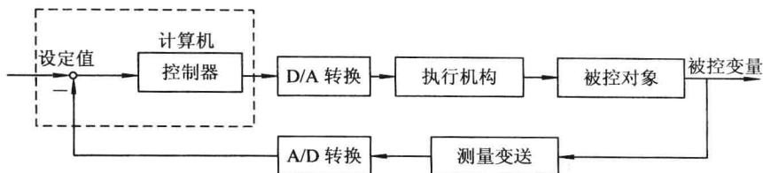
图 1-1-1 计算机闭环控制系统结构框图
