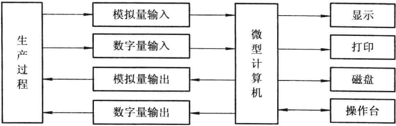
图 1-1-4 直接数字控制系统结构图
