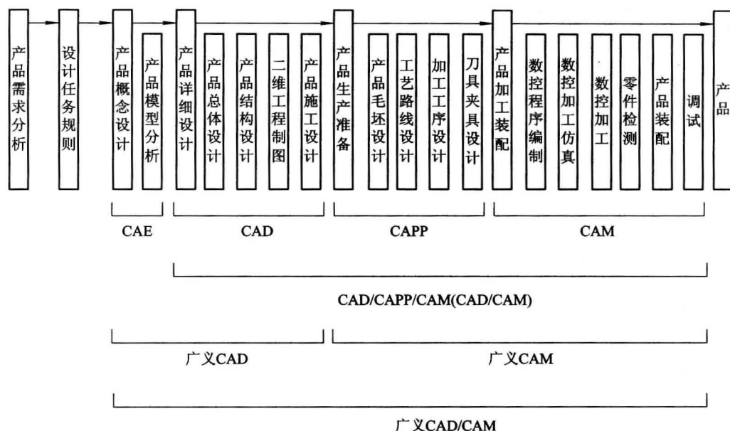
图 1.1.1 产品开发过程及 CAD、CAE、CAM 的范围
