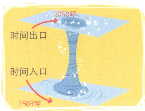
时空隧道假想图
