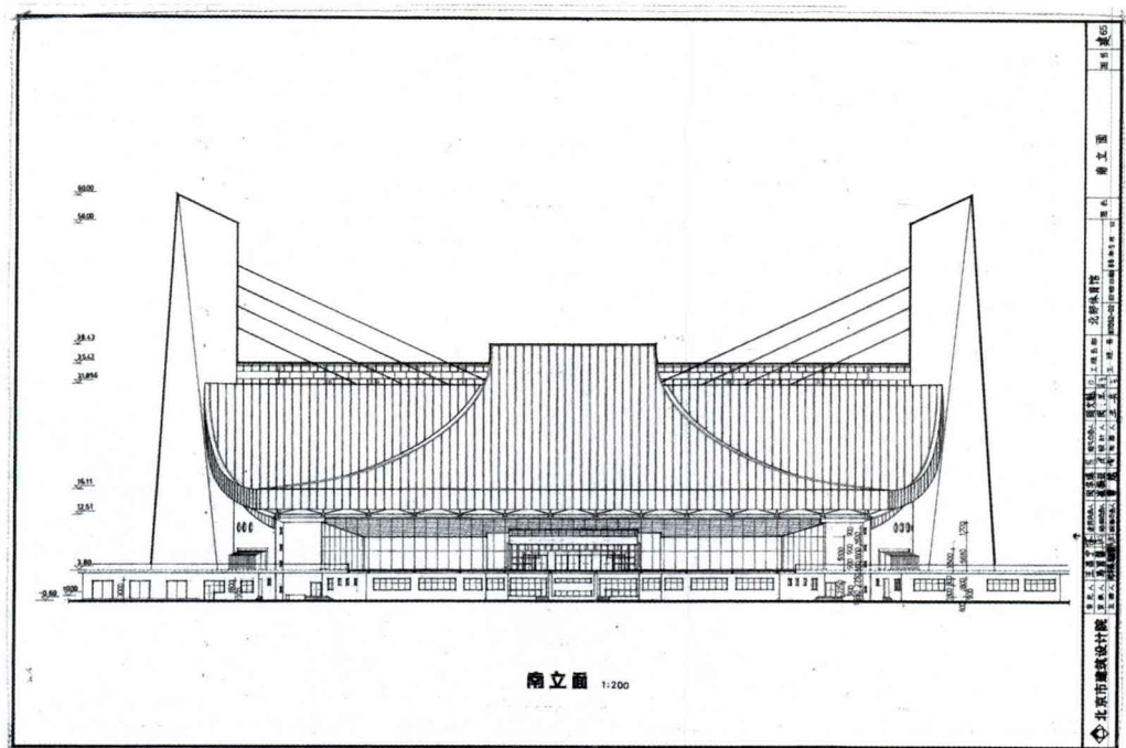
图3 1988年王兵绘制的亚运体育馆立面图
