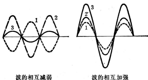
图 1-1-1 波的干涉
