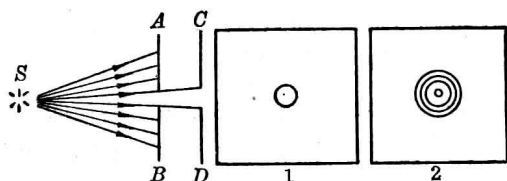
1. 圆孔较大时在屏上得到的光亮圆; 2. 圆孔很小时在屏上得到的衍射环。
