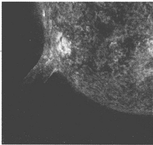
太阳风
