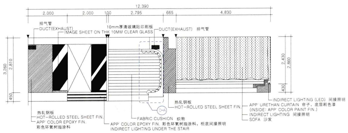
Elevation D D立面
