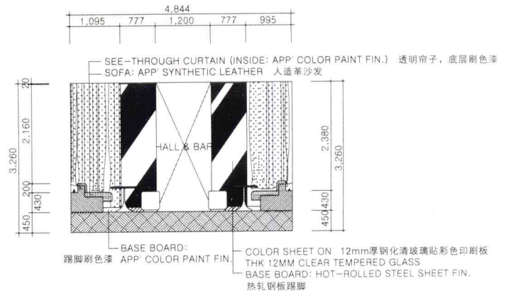
Elevation F F立面
