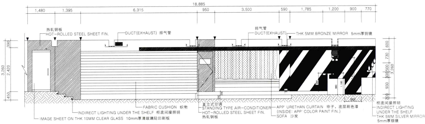
Elevation C C立面
