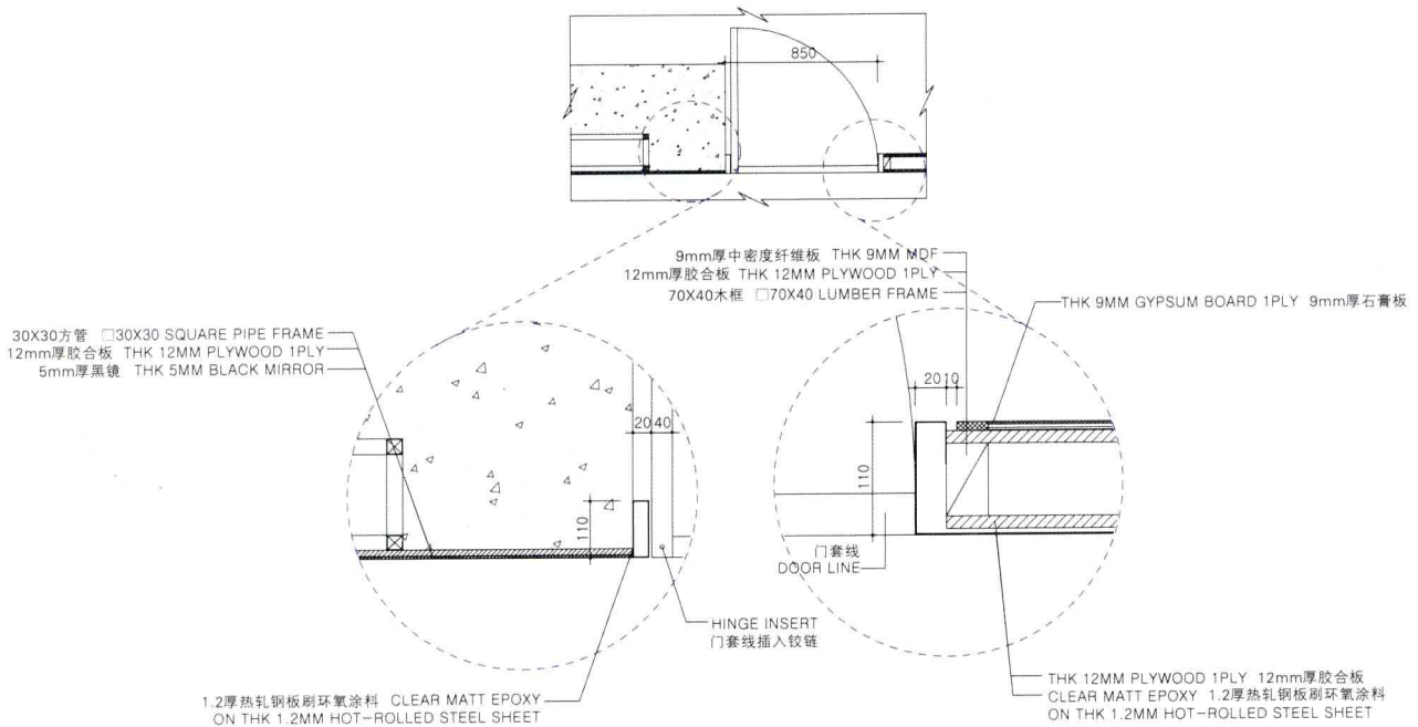
Section B B剖面
