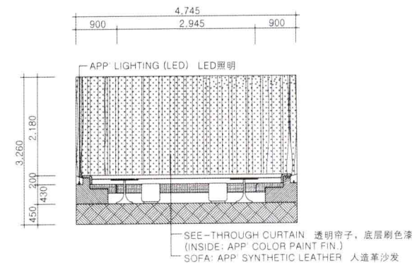
Elevation H H立面
