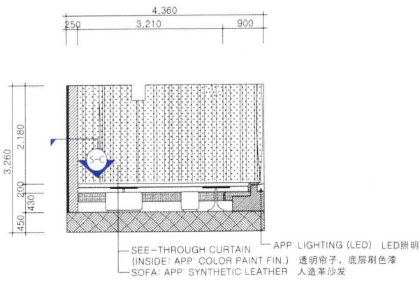
Elevation E E立面
