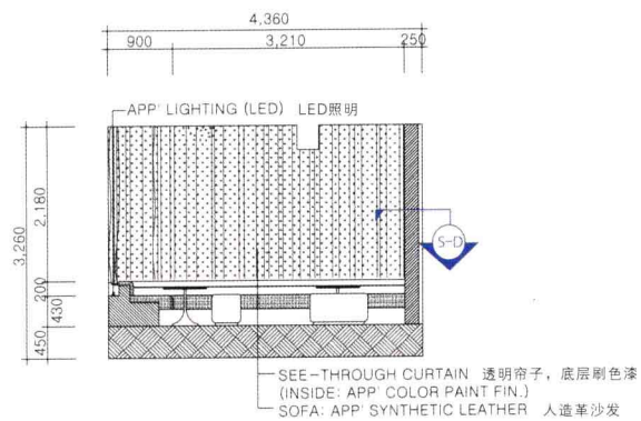
Elevation G G立面
