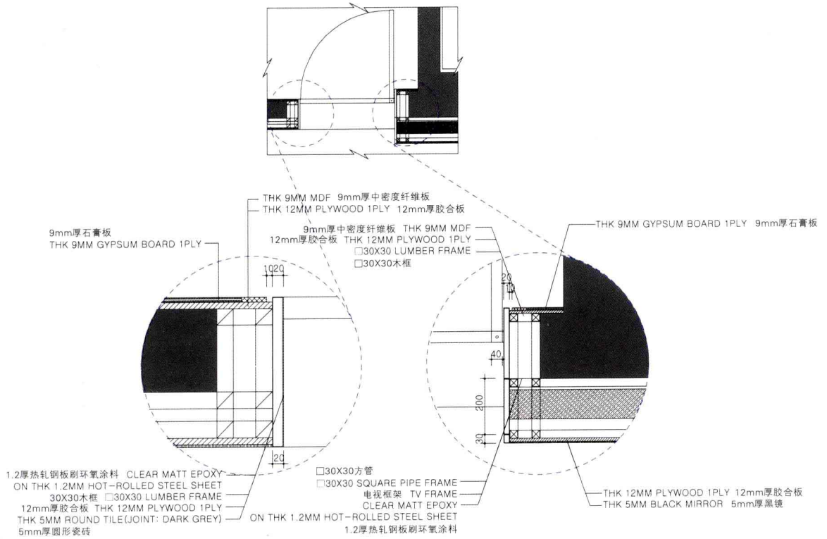
Section A A剖面
