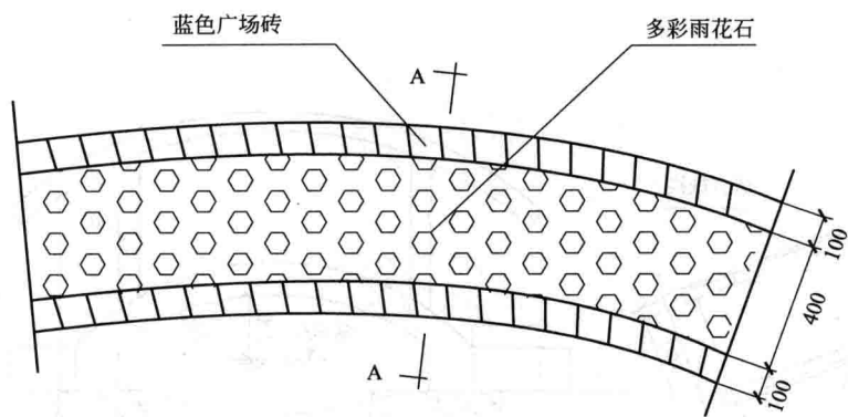
① 休闲小径示意图
