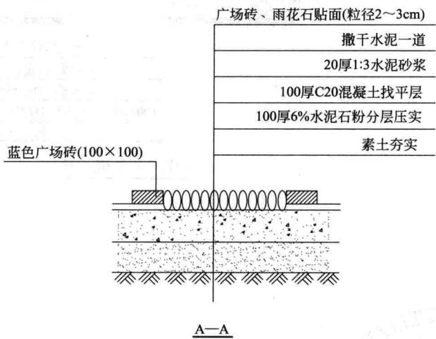
① 休闲小径示意图
