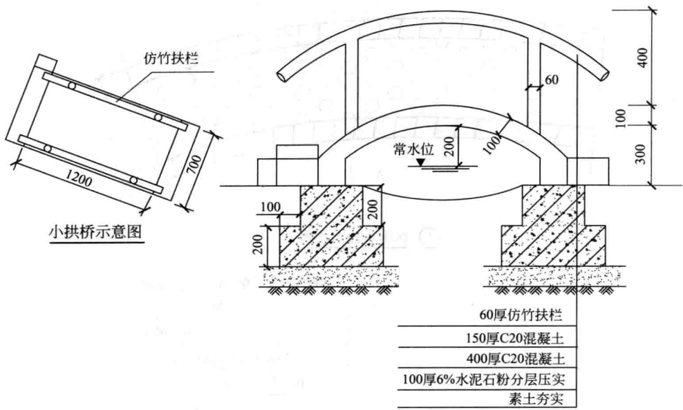
仿竹小拱桥施工图
