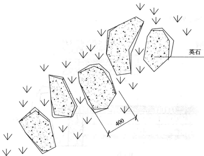
英石嵌草踏步施工图
