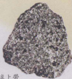
从月球上带回的岩石
