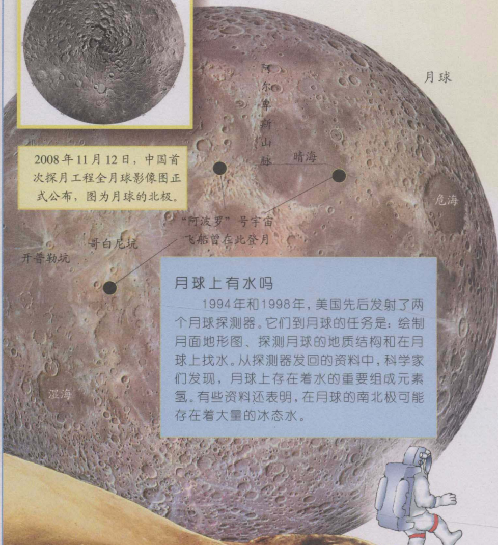
月球表面景观
