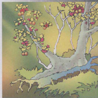
北半球秋天 南半球春天
