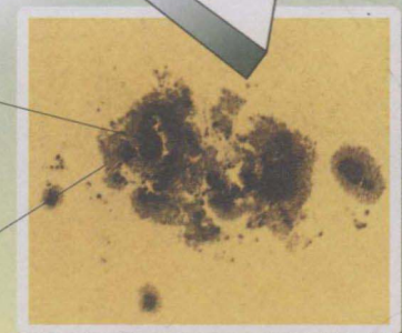
中间较暗的部分为黑子的本影
