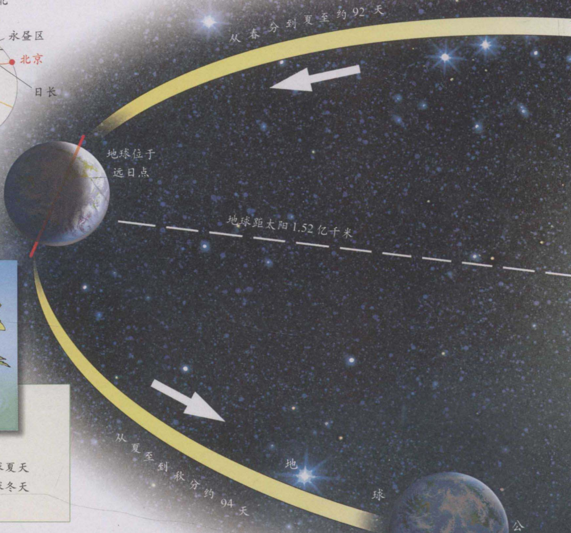
夏至(6月22日前后)
