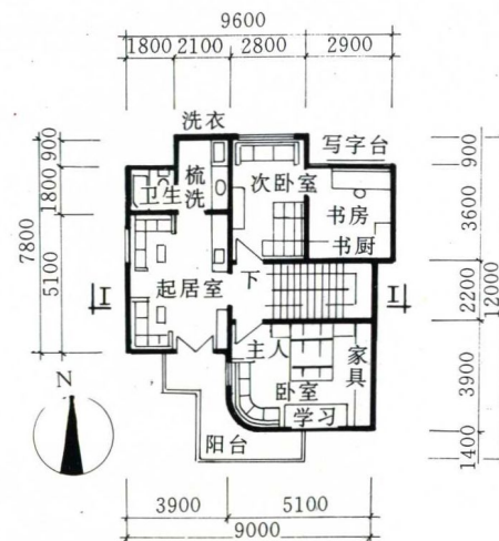
二层平面图
