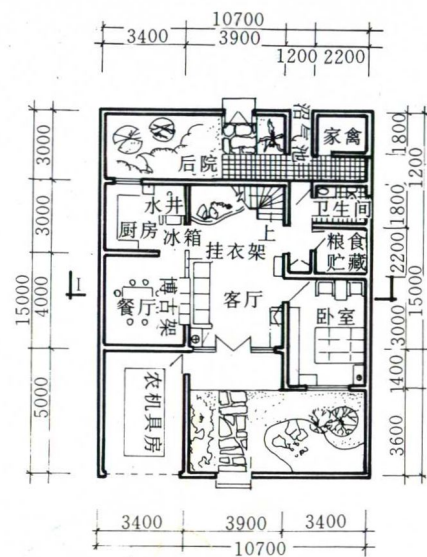
底层平面图
