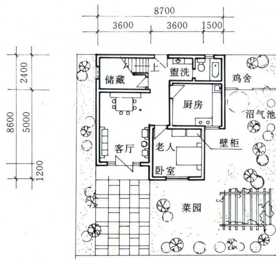
一层平面图
