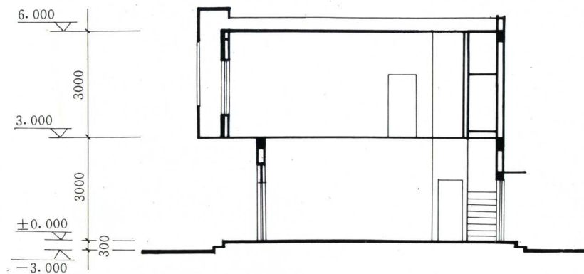
剖面图
