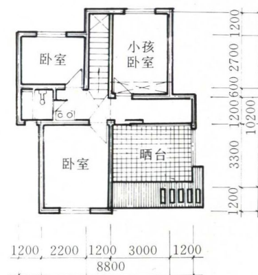
二层平面图
