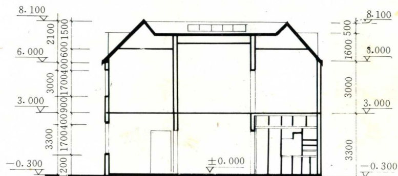
I-I 剖面图
