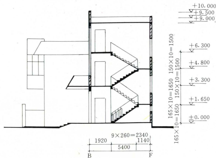
楼梯剖面图
