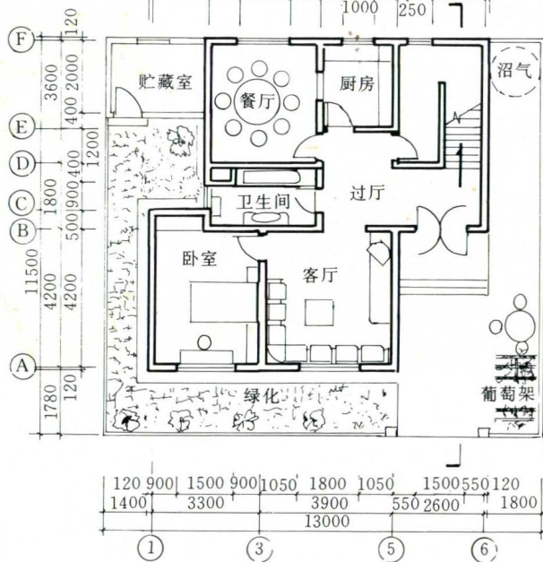
底层平面图
