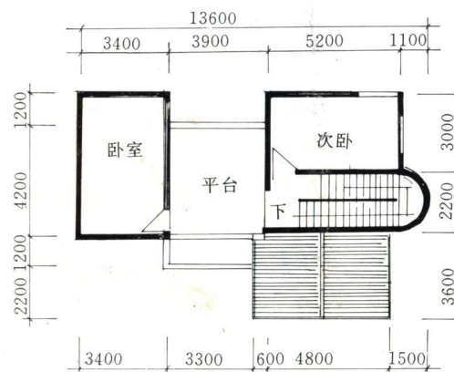
三层平面图
