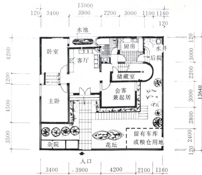
底层平面图
