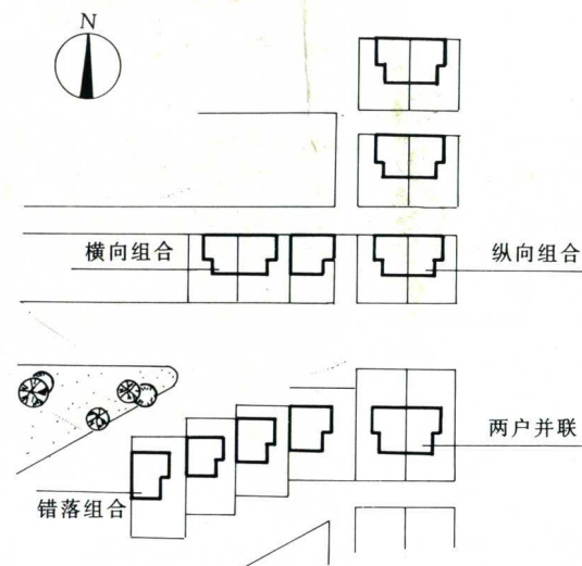
平面组合示意图
