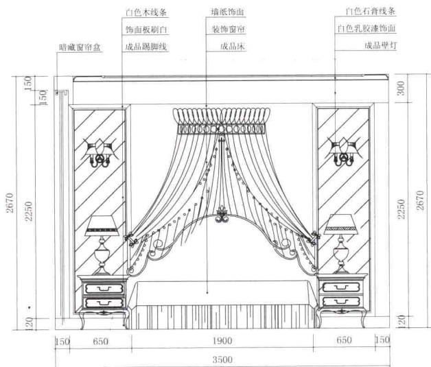
床背景立面图
