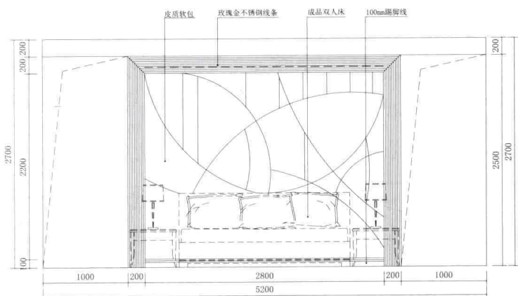
床背景立面图
