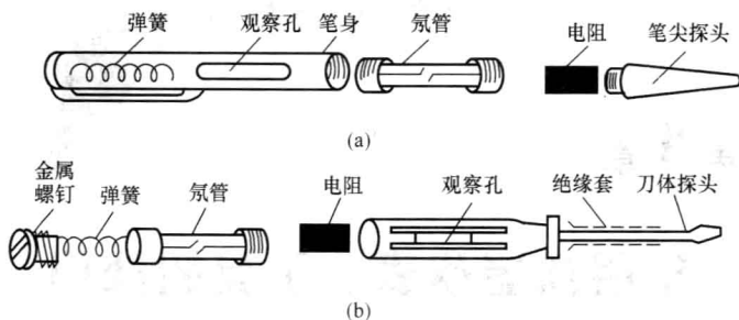
图 1-1 低压验电器
