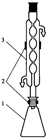
图 1.2 重结晶回流装置
