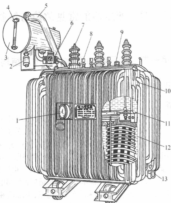
图 1-1 油浸式电力变压器
