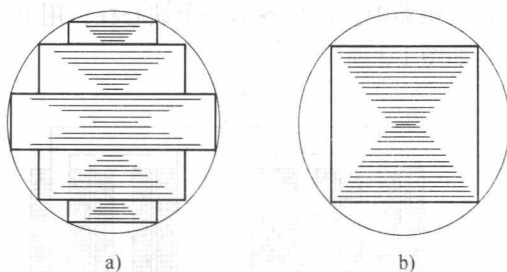
图 1-5 铁心柱截面
