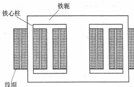
图 1-3 三相心式变压器
