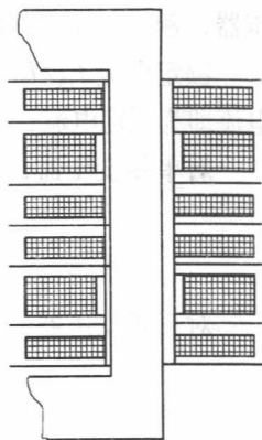
图 1-6 高低压绕组互相交叠放置
