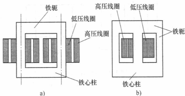
图 1-2 单相变压器的基本形式
