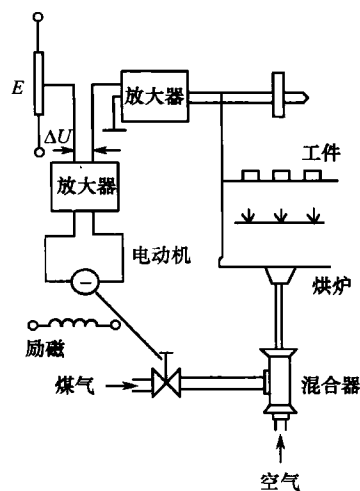
图 1-16 烘烤炉温度控制系统
