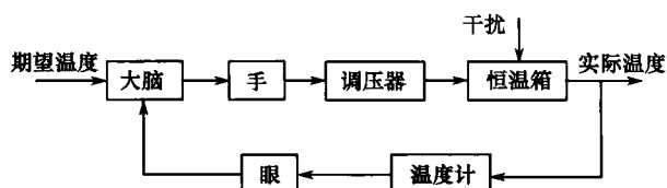
图 1-2 人工控制职能图
