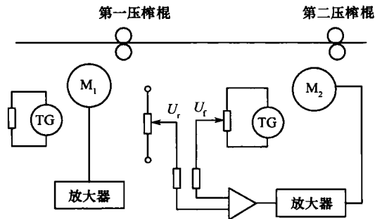
图 1-14 造纸机分部传动控制系统原理图
