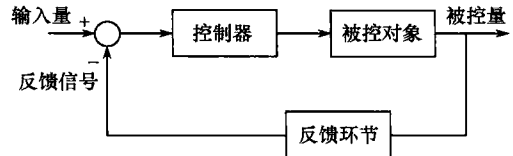
图 1-9 闭环控制系统方框图
