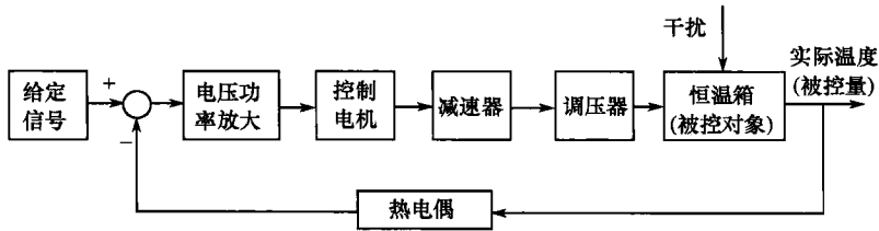
图 1-4 恒温箱自动控制系统信号流程图
