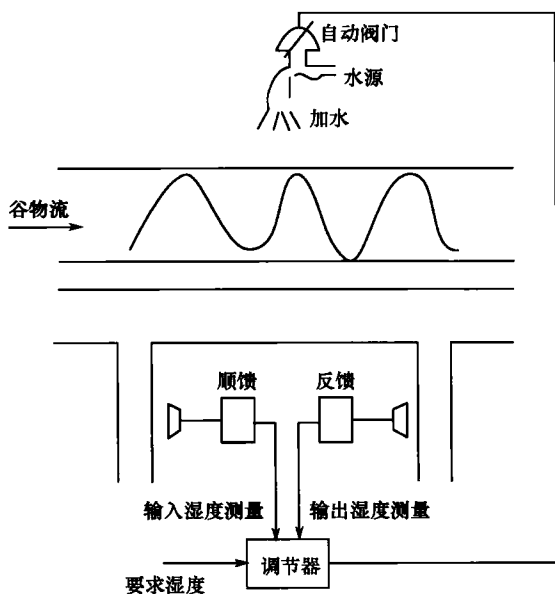
图 1-15 谷物湿度控制系统
