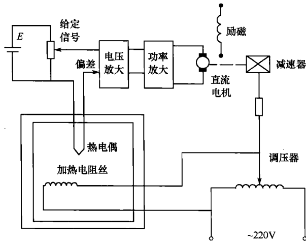
图 1-3 恒温箱自动控制系统示意图
