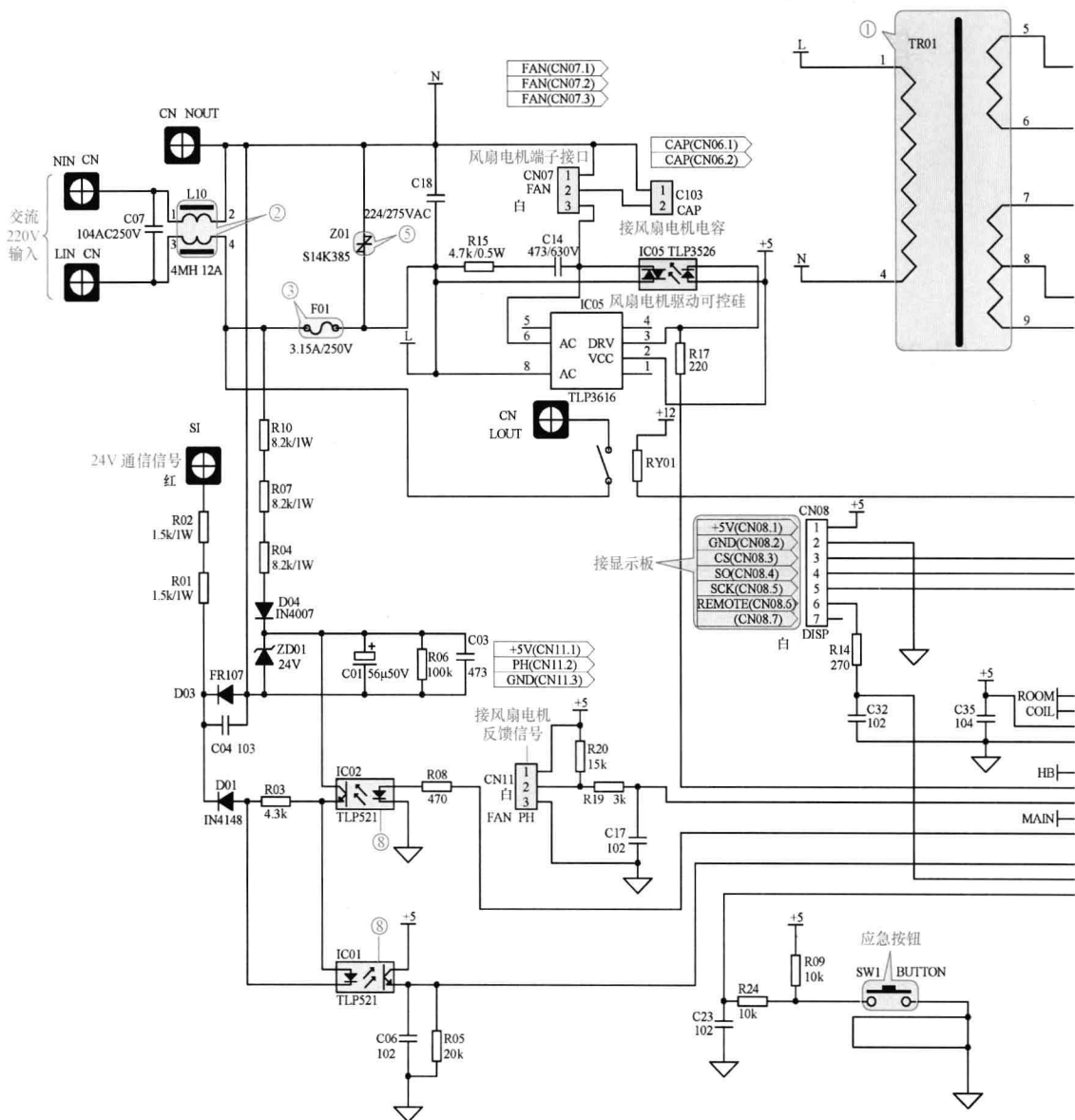
2. KFR-26GW/77ZBp 系列空调器室内机控制板电路原理图
