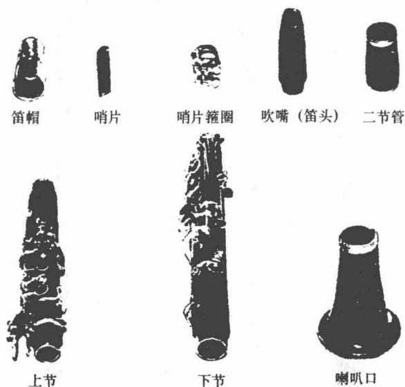
图 1-2 单簧管各部件名称
