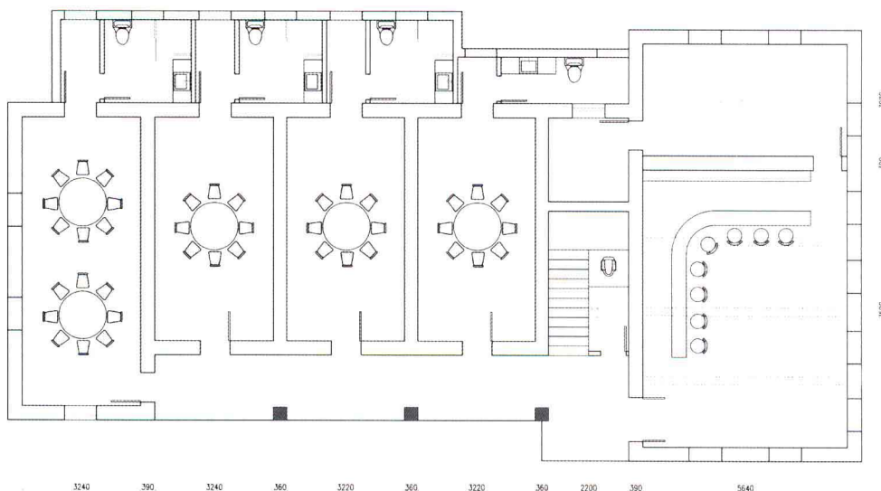
一层平面图
