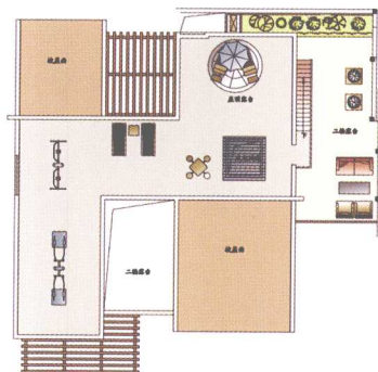
顶层平面图
