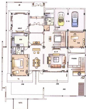
一层平面图
