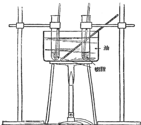
圖 6 酚甲醛树脂(一級反应的酚甲醛树脂及諾复腊型酚甲醛树脂)对热的影响。在油浴鍋中加熱
