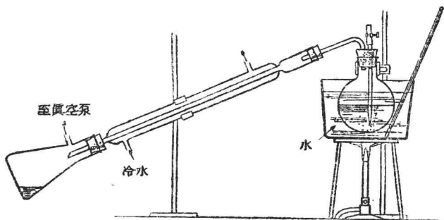
圖 5 真空蒸溜。在迴流中所形成的水分，用低溫真空管蒸餾除去，以免樹脂太老
