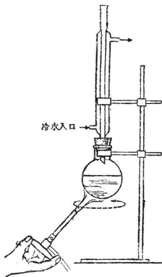
圖2 迴流裝置。燒瓶 上有裝有迴流冷凝管
