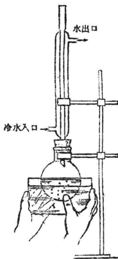
圖3 減緩放热反 应的方法
