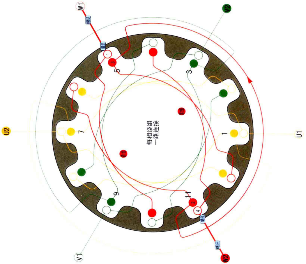
b) 接线图
