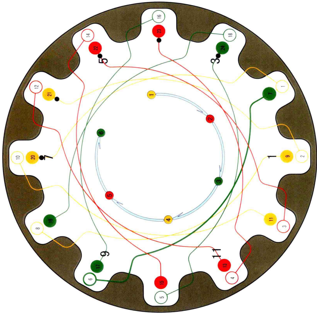
a) 嵌线图
