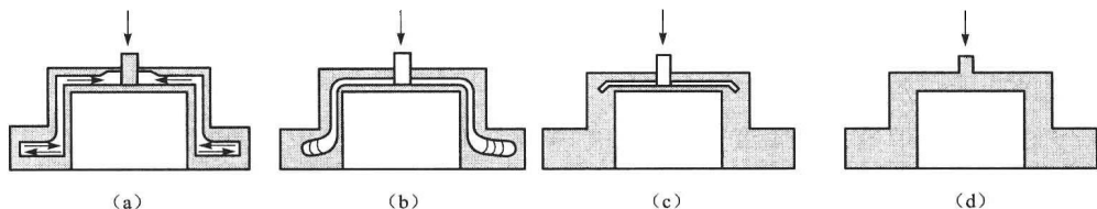
图1-5 三阶段充填理论的充填形态
