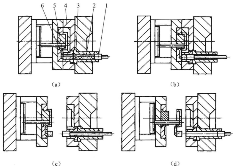
图 1-1 金属压铸成形
