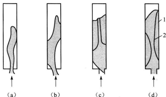
图 1-8 薄壁型腔充填形态
