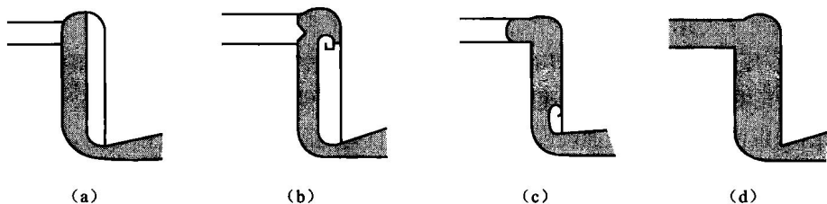
图 1-9 金属流在型腔转角处的充填形态
