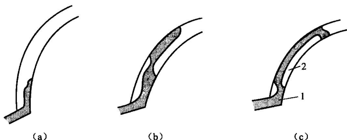
图 1-10 金属液在圆弧面处的充填形态
