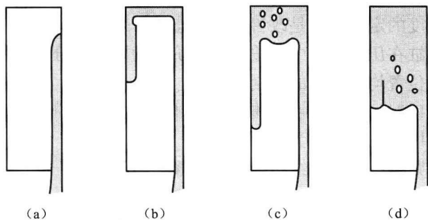
图 1-7 内浇口在型腔一侧时的充填形态
