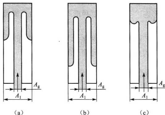
图 1-6 不同内浇口截面积厚度的充填形态
