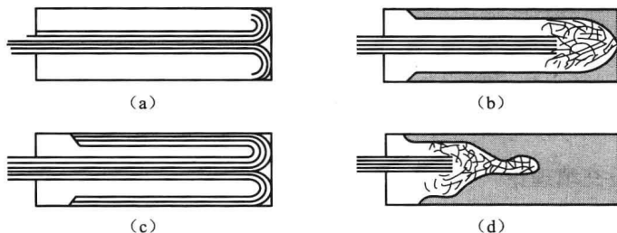
图1-3 金属液在型腔内的充填形态
