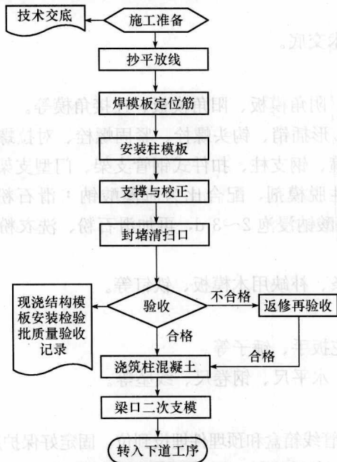
图 1-6 柱模板安装施工工艺流程
