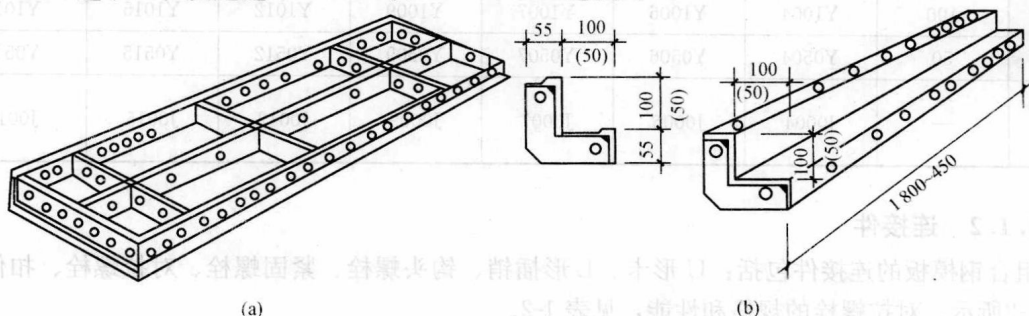
图 1-1 钢模板的类型 (一)
