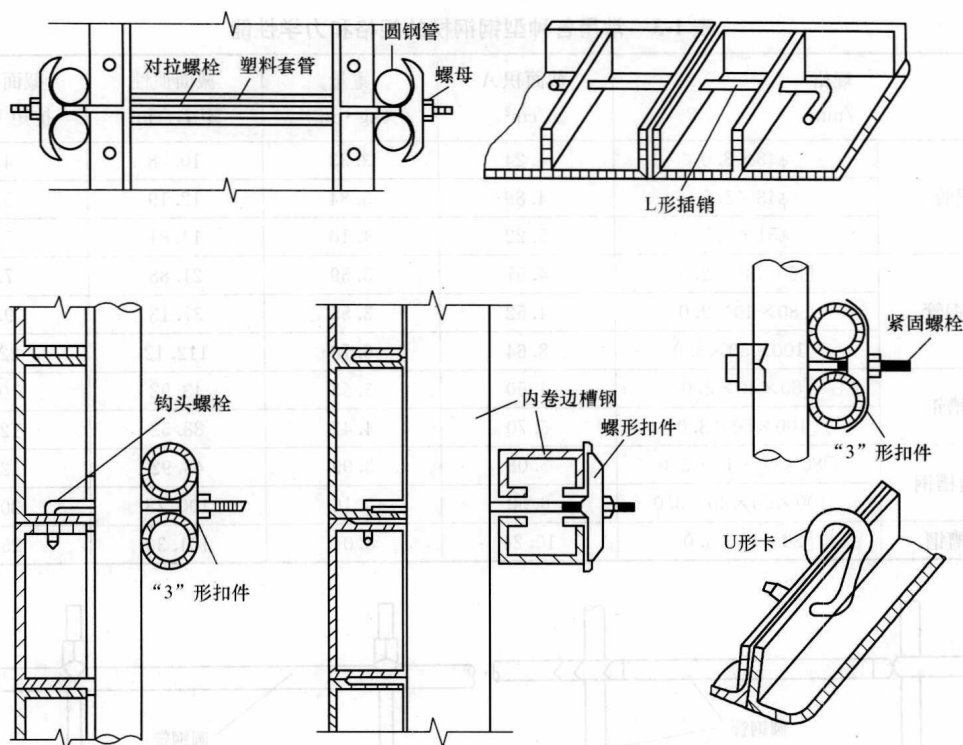
图 1-2 钢模板连接件
