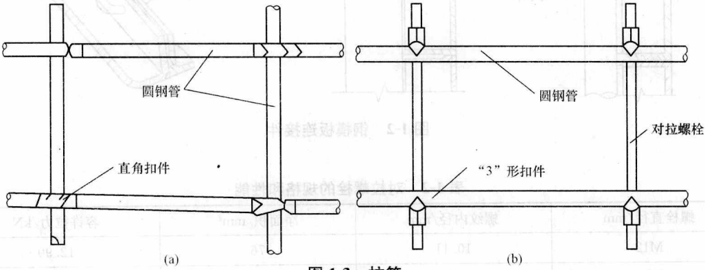
图 1-3 柱箍
