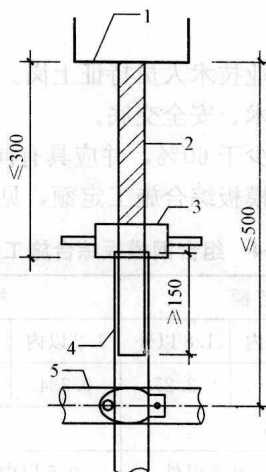
图 1-5 支架顶部构造
