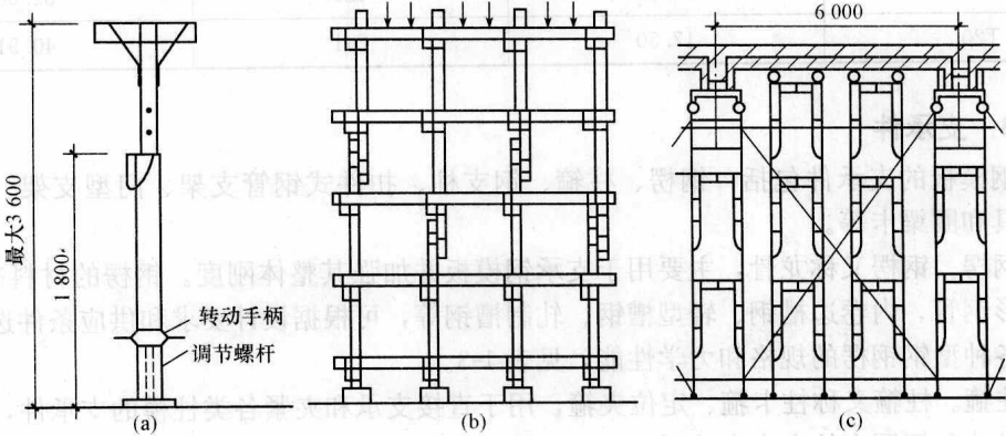
图 1-4 钢支柱柱箍
