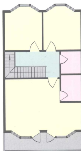
二层平面图
