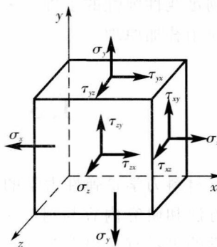
图 1-4 体元素上应力分量
