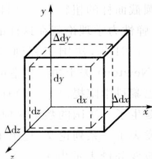
图 1-5 体元素的变形
