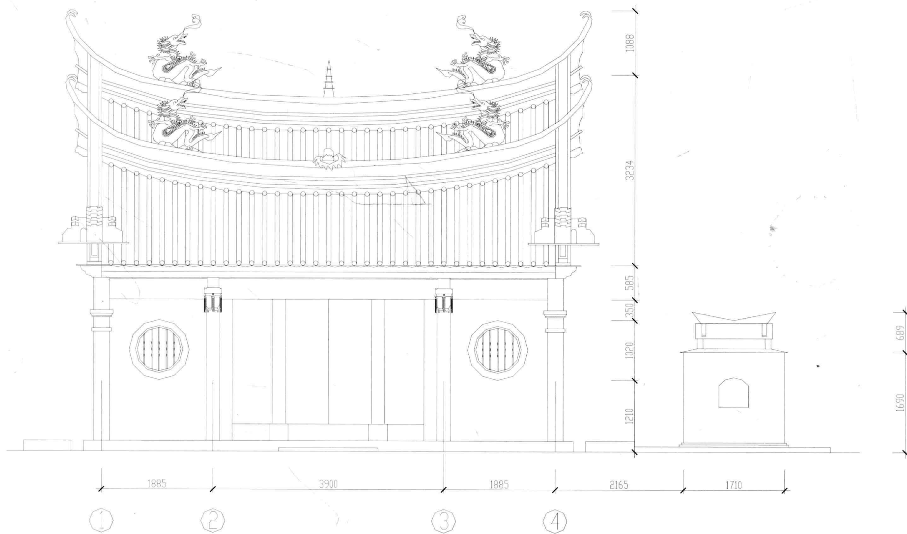
正立面图
