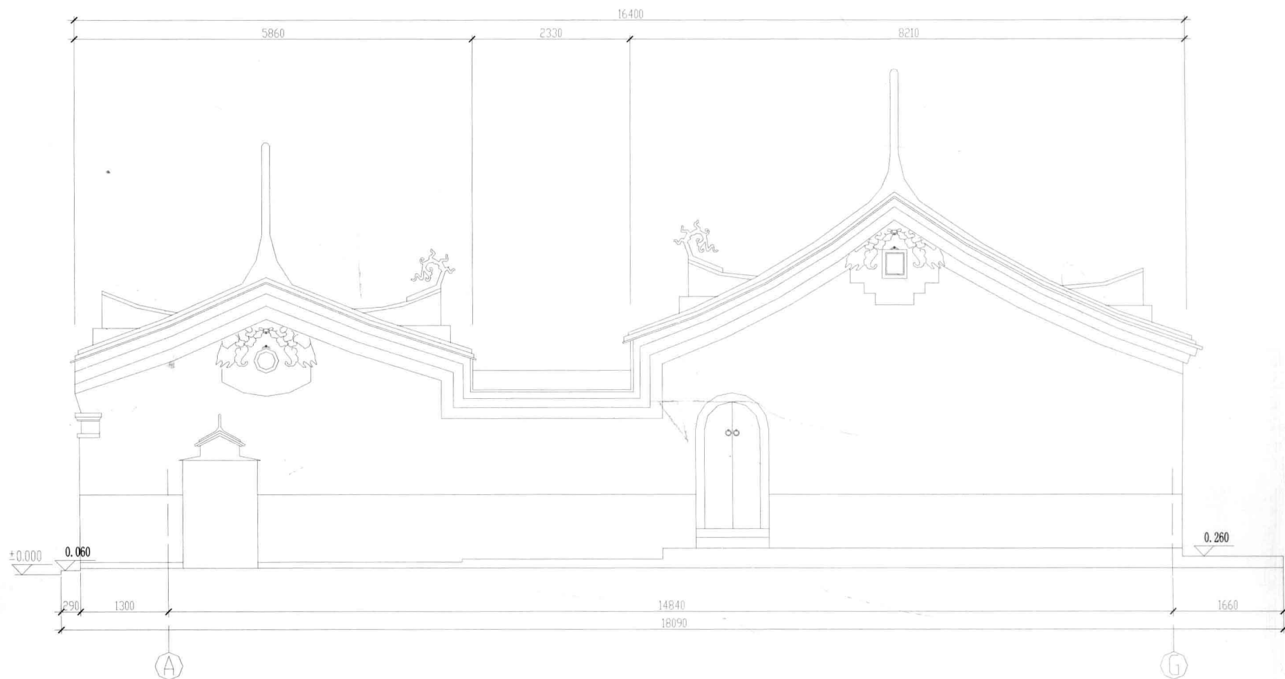
侧立面图
